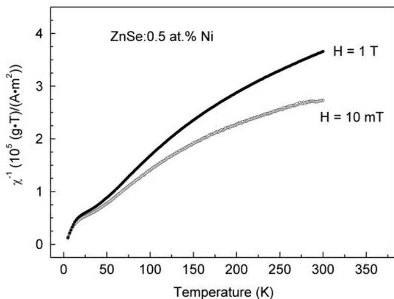
Fig. 2. Influența intensității câmpului magnetic asupra dependenței de temperatură a susceptibilității magnetice inverse a cristalului de ZnSe:0,5% at. Ni.
