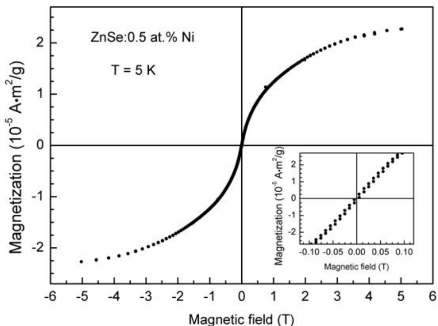
Fig. 3. Cercetarea histerezisului magnetic pentru cristalul de ZnSe:0,5% at. Ni.
