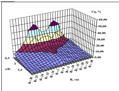
Fig. 3. Diagrama tridimensională a câmpului concentrației gazului pentru arzător cu stabilizator tip C la P_{max} , D_c=124\text{mm} .
