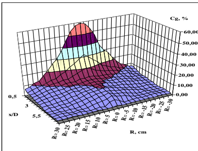
Fig. 2. Diagrama tridimensională a câmpului concentrației gazului pentru arzător cu stabilizator tip B la P_{min} , D_c=124\text{mm} .
