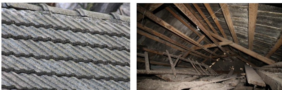
Figura A3.4.3. Acoperiș în 2 pante cu oale din cement. Construcția de susținere a acoperișului în 2 pante (aspectul din interior), foto autor, 2018. S. Stoianovca, raionul Cantemir
