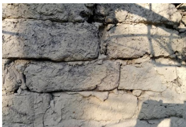
Figura A3.3.4. Pereți de casă ridicate cu lampaci (chirpici nears), unse cu 2 straturi de lut și date cu var, foto autor, ianuarie 2018. S. Stoianovca, raionul Cantemir
