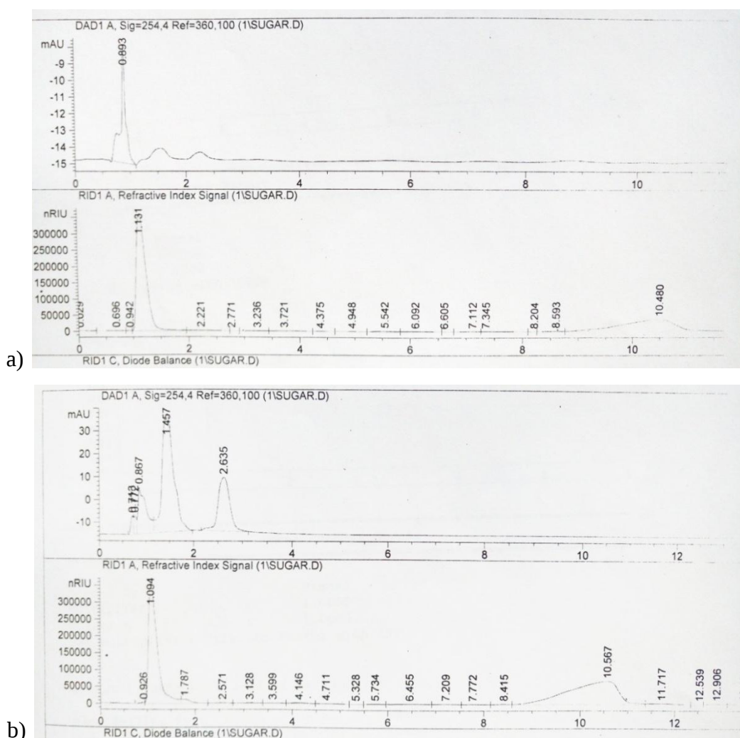
Fig. 4.3. Cromatografie lichidă (HPLC): a) Cromatograma soluției standard de lactoză; b) Cromatograma probei de lapte de capră-materie primă (Autorul foto Bogdan N.)
