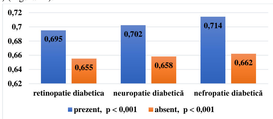
Figura 13. IRR în funcție de prezența disglucemiei și a complicațiilor microvasculare în lotul pacienților cu DZ
