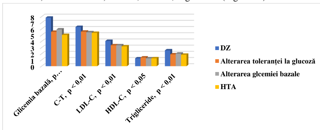
Figura 11. Particularitățile profilului lipidic și glucidic la pacienții din loturile de cercetare.
