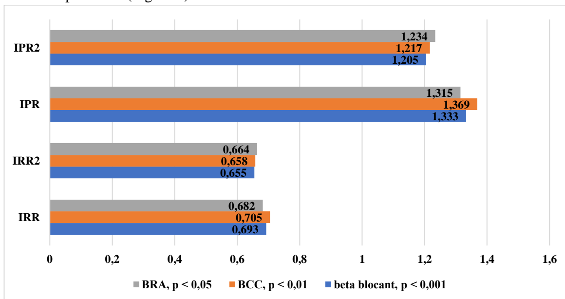
Figura 3. Variațiile parametrilor HIR în funcție de tratamentul antihipertensiv administrat
