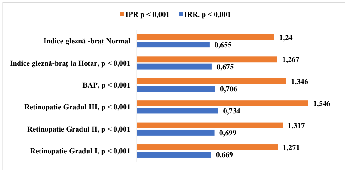
Figura 4. Corelațiile parametrilor HIR cu afectarea vasculară periferică și retinopatia la pacienții hipertensivi
