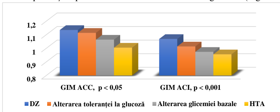
Figura 12. Particularitățile GIM în dependență de prezența disglucemiei și tipurile acesteia.
