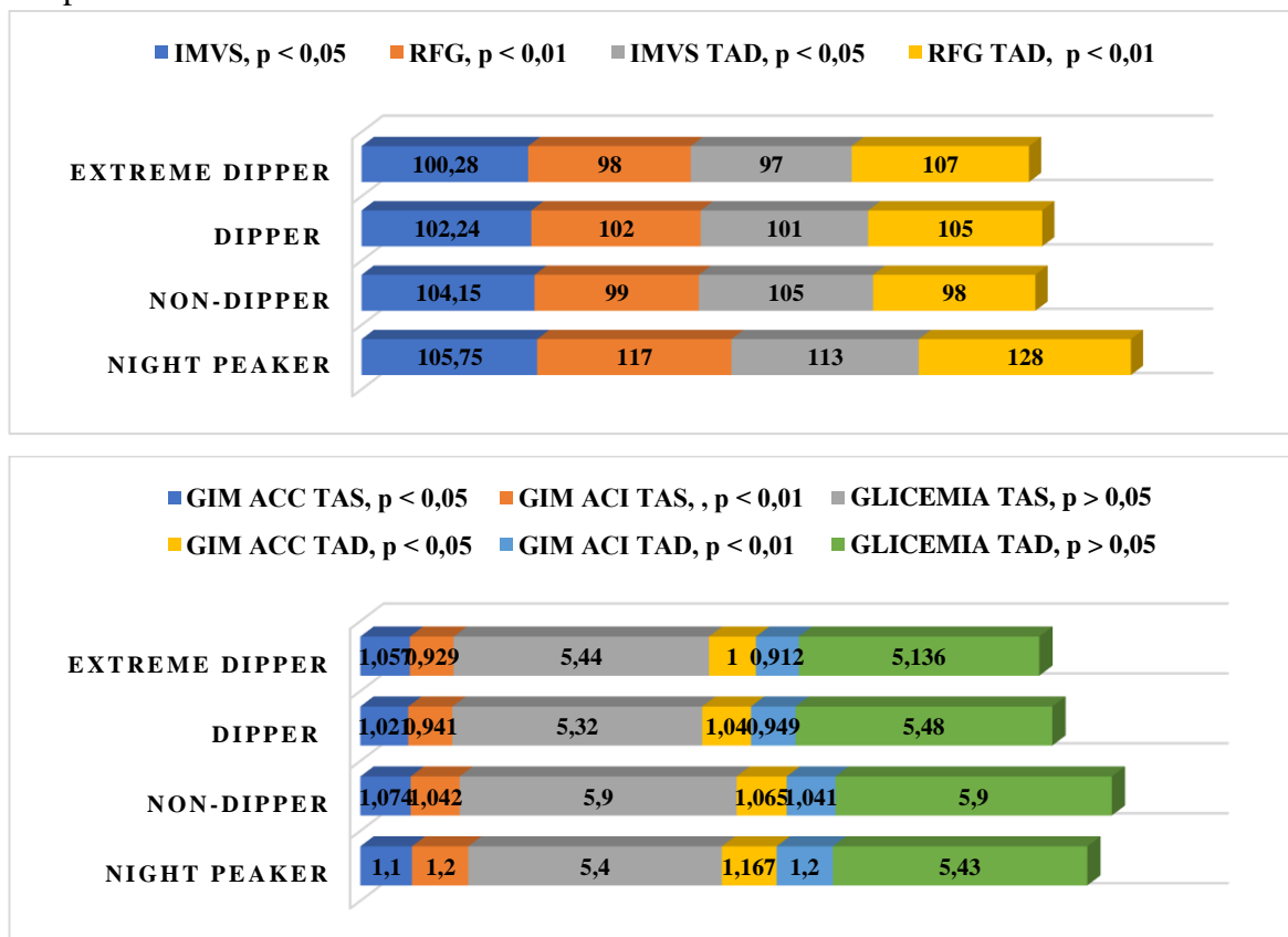
Figura 9. Analiza comparativă a modelelor variației nictimerale a TAS și TAD cu parametrii AAOȚ și glicemia bazală.
