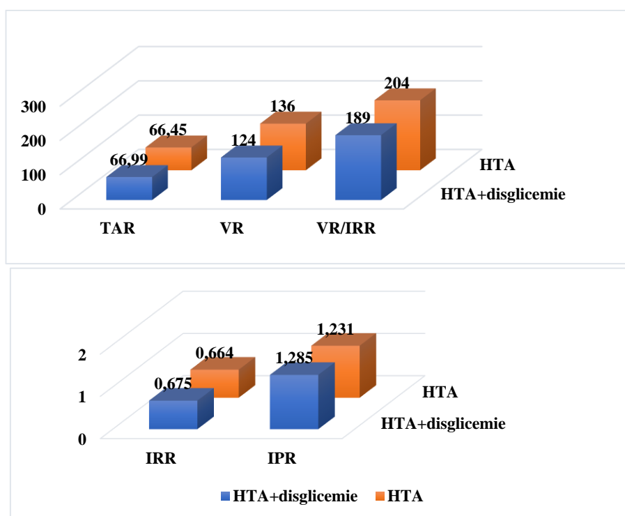
Figura 10. Diferențele variabilelor HIR în funcție de prezența disglicemiei.
