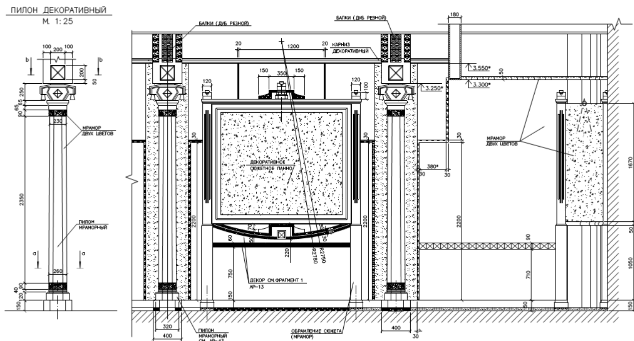
Figura A3.31. „Sala Prezidențială”. Fragment al desfășurării peretelui longitudinal
