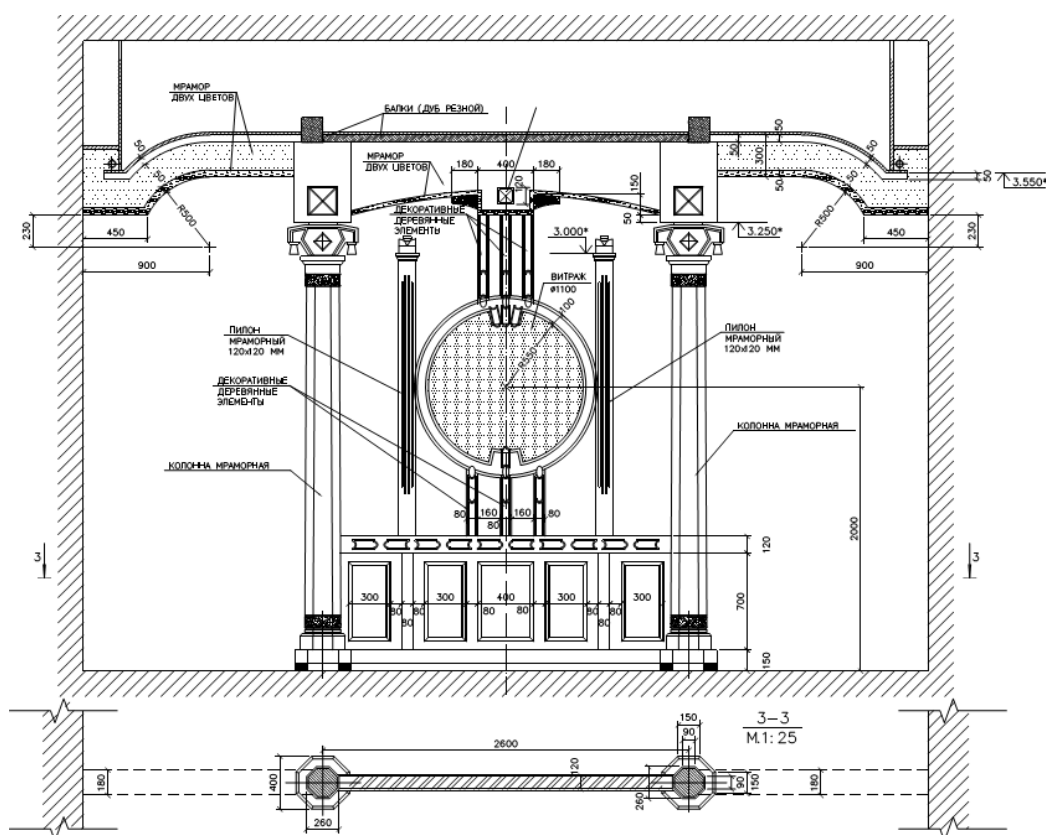
Figura A3.32. „Sala Prezidențială”. Perete despărțitor decorativ
