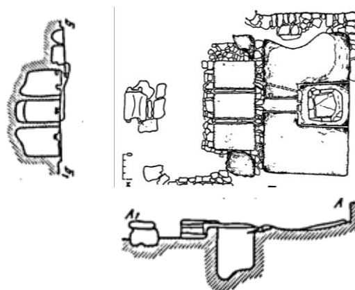
Figura A2.4. Planul, secțiunile și reconstituirea cramei cu trei rezervoare din Tyritake , sec. III-IV p.Chr. (după Kruglikova, 1984)
