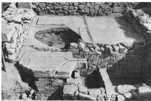
Figura A2.2. Crama cu două compartimente ale rezerveului din Mirmekion , sf. sec. III a.Chr. (după Блаватский, 1953)
