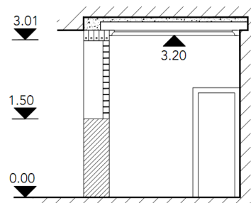
Figura A2.41. Secțiune 2-2
