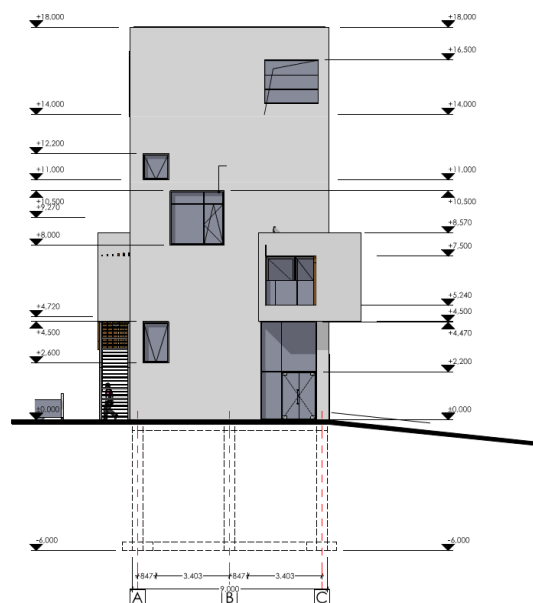
Figura A4.85. Fațada în axele A-C
