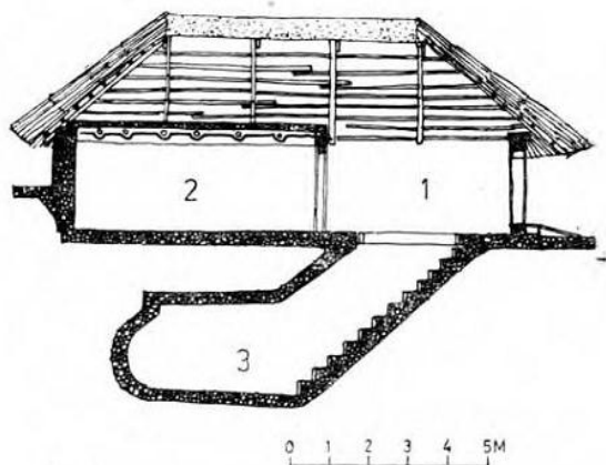
Figura A2.8. Cramă de vie din Corni, județul Vaslui. Mijl. sec. XIX. Secțiune: 1 – horă; 2 – cramă; 3 – beci. (după Patrașcu, 1984)
