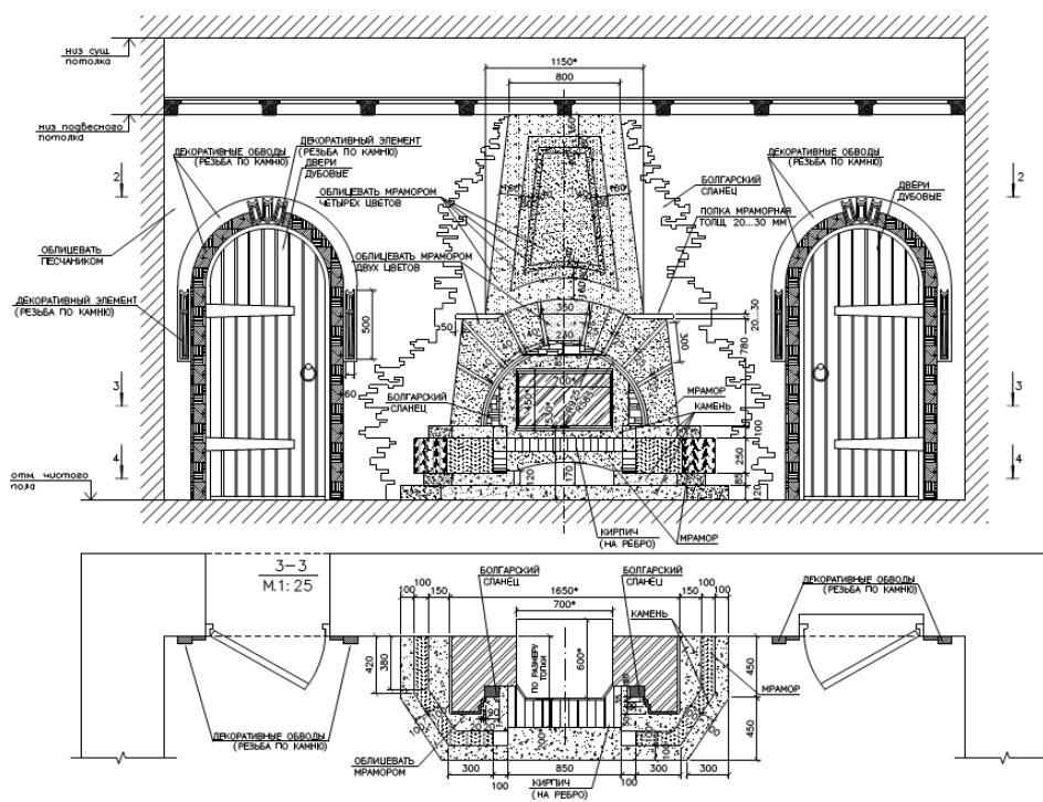
Figura A3.36. Sala cu șemineu. Fragment al desfășurării peretelui latitudinal
