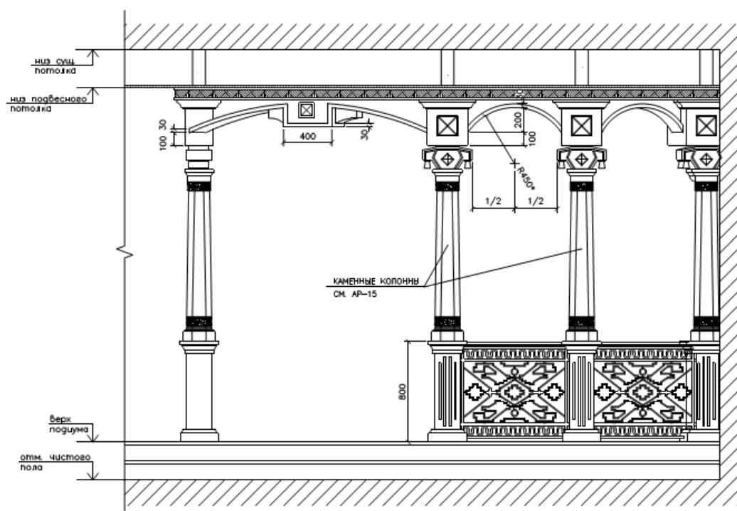
Figura A3.41. Holul central. Fragment semirotondă
