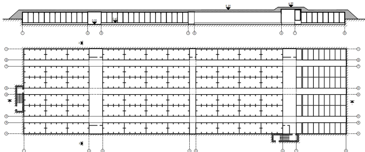
Figura A2.32. Secțiunea 1-1 și planul depozitului de vinuri
