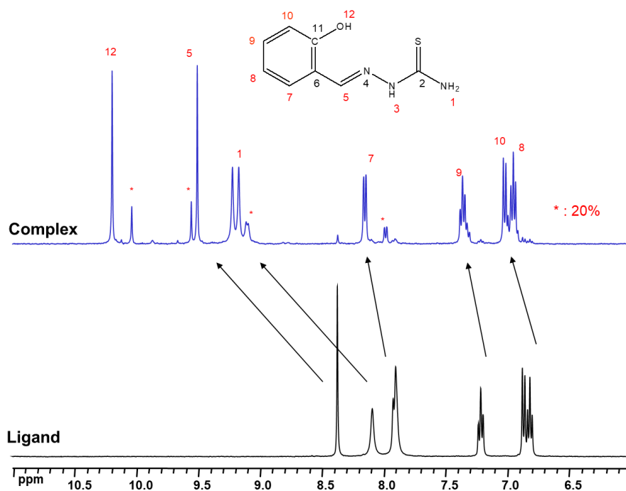
Fig. 3.2. Analiza ^1\text{H} RMN a ligandului și compusului [\text{Mo}_2\text{O}_2\text{S}_2(\text{C}_8\text{H}_8\text{N}_3\text{SO})_2] [29]
