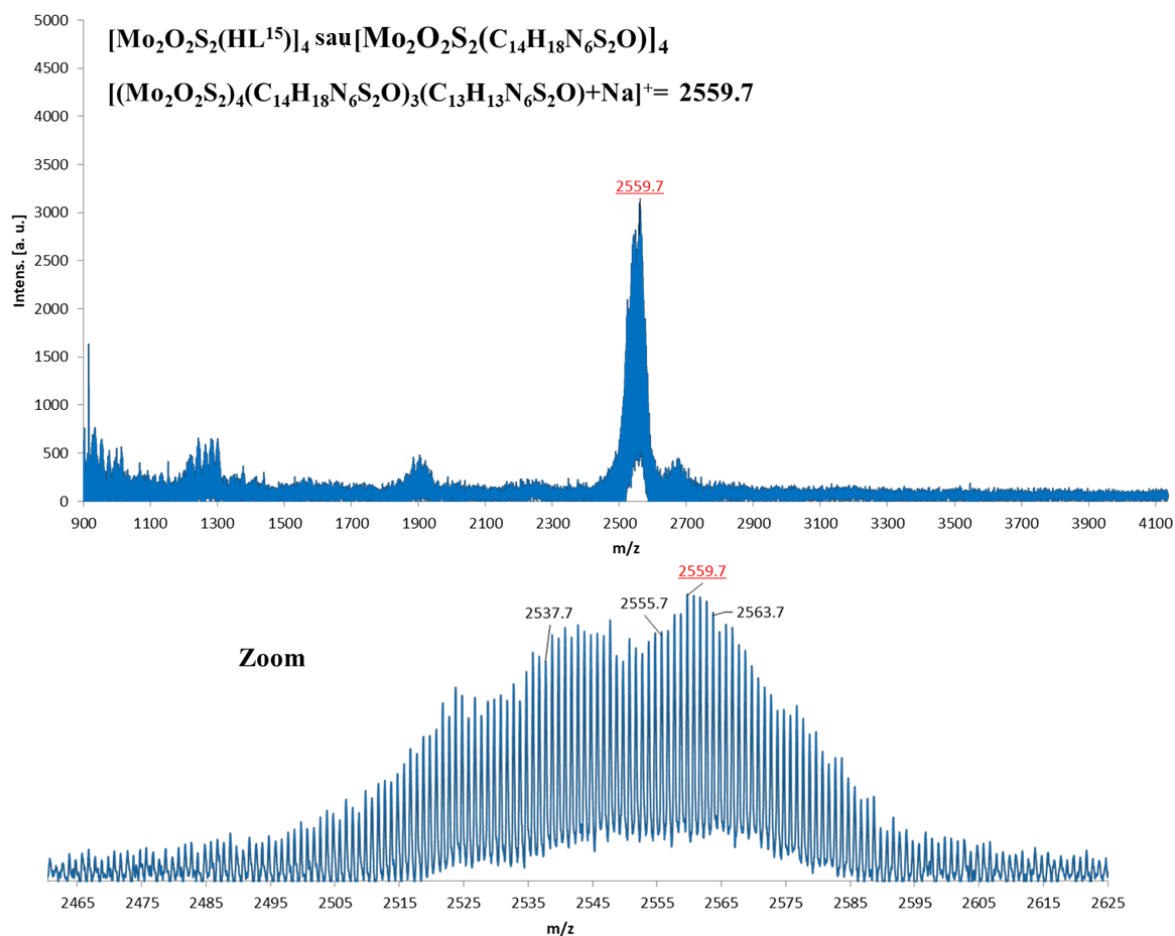
Fig. A6.8 Spectru de masă MALDI-TOF al compusului [Mo_2O_2S_2(HL^{15})]_4
