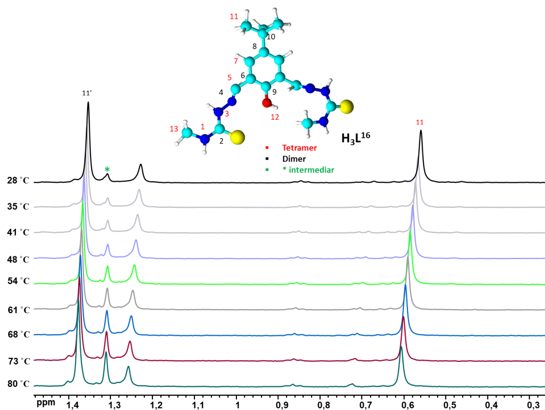
Fig. A8.9 400 MHz ^1\text{H} RMN (DMSO- \text{d}_6 ) spectru al complexului [\text{Mo}_2\text{O}_2\text{S}_2(\text{HL}^{16})]_2 și [\text{Mo}_2\text{O}_2\text{S}_2(\text{HL}^{16})]_4 la diferite temperaturi (de la 28 la 80 °C)
