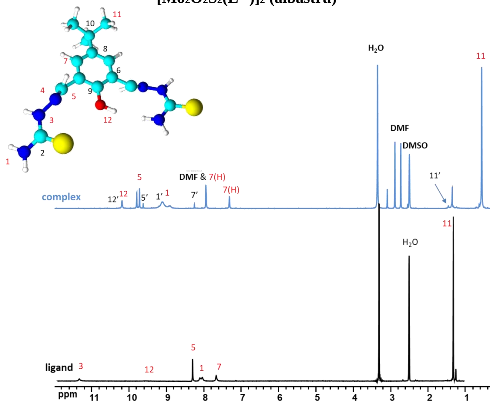
Fig. A8.8 400 MHz ^1H RMN (DMSO- d_6 ) spectru al ligandului H_3L^{15} (negru) și al complexului [Mo_2O_2S_2(HL^{15})]_2 și [Mo_2O_2S_2(HL^{15})]_4 (albastru)
