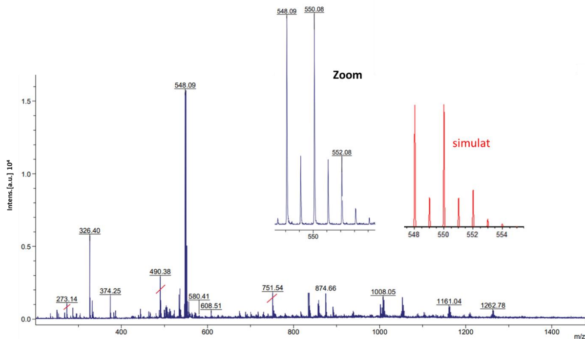
Fig. 4.32. Spectrul de masă MALDI-TOF al compusului [\text{Cu}_2(\text{L}^{16})\text{OC}_2\text{H}_5]
