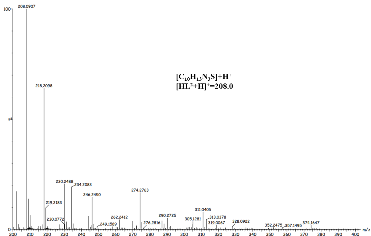
Fig. A2.2 Spectru de masă ESI-MS al mono-tiosemicarbazonei HL 2
