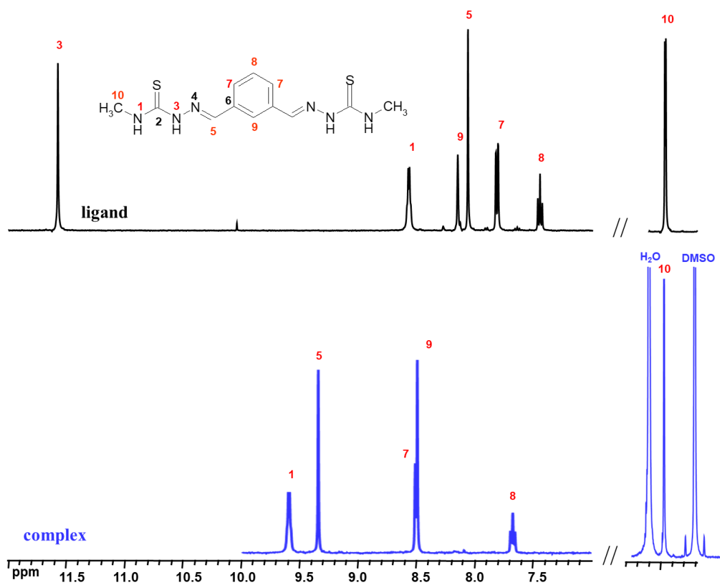
Fig. A8.7 400 MHz ^1H RMN (DMSO- d_6 ) spectru al ligandului H_2L^{14} (negru) și al [Mo_2O_2S_2(L^{14})]_2 (albastru)
