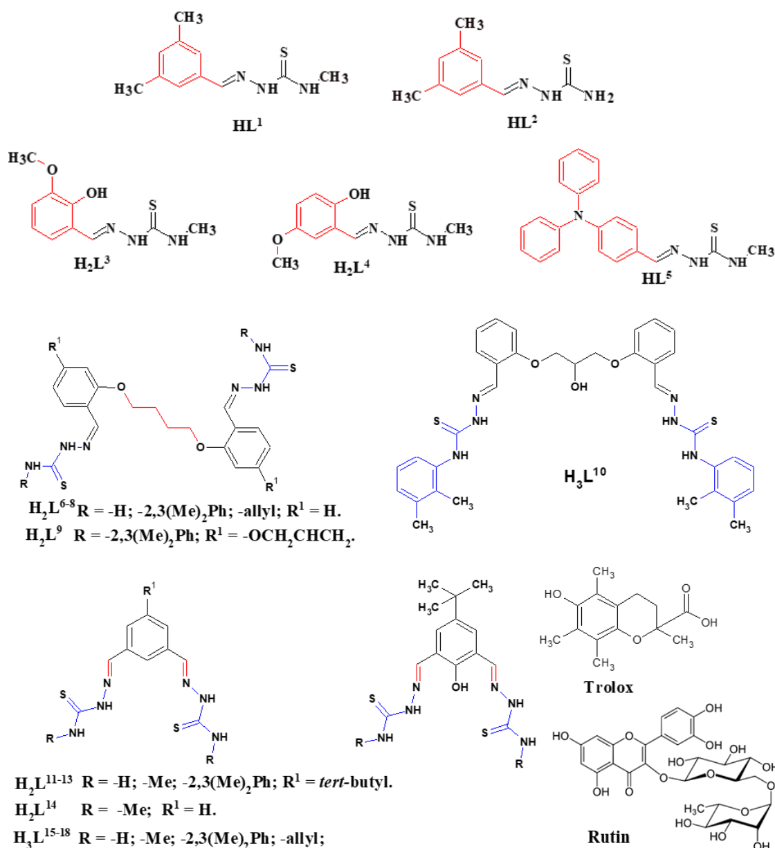
Fig. 5.1. Structurile liganzilor sintetizați și referințelor: Trolox și Rutin
