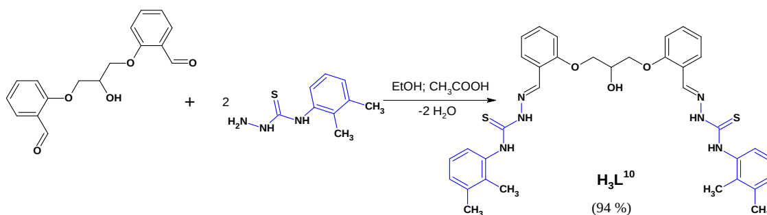
Fig. 2.4. Schema de sinteză a bis-tiosemicarbazonei H 3 L 10
