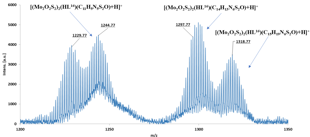
Fig. 4.18. Zoom - spectrul de masă MALDI-TOF al compusului [Mo_2O_2S_2(HL^{16})]_4
