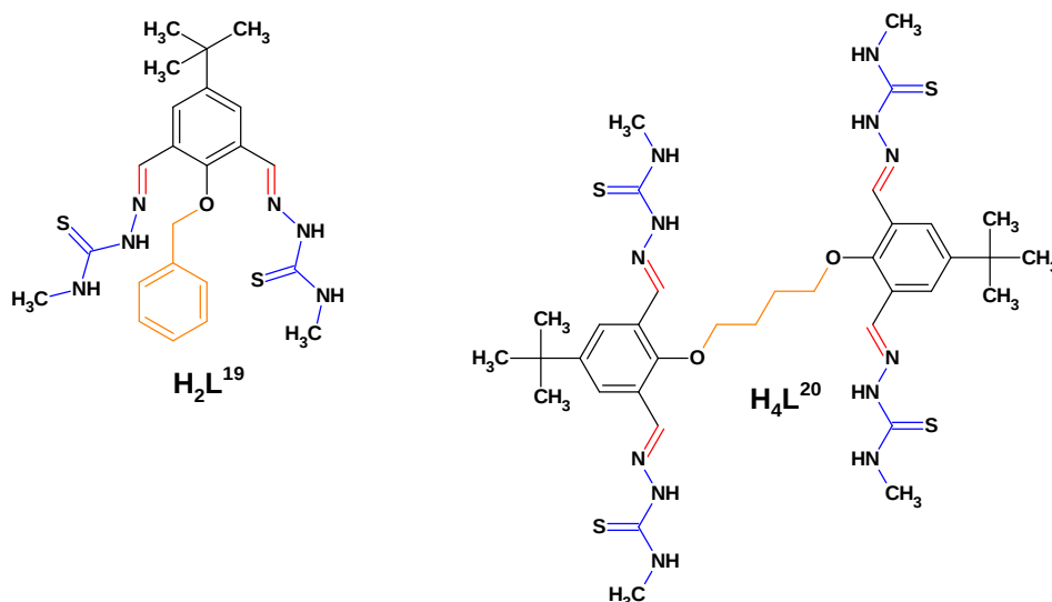
Fig. 4.27. Structurile chimice ale bis-tiosemicarbazonei H 2 L 19 și tetrakis-tiosemicarbazonei H 4 L 20
