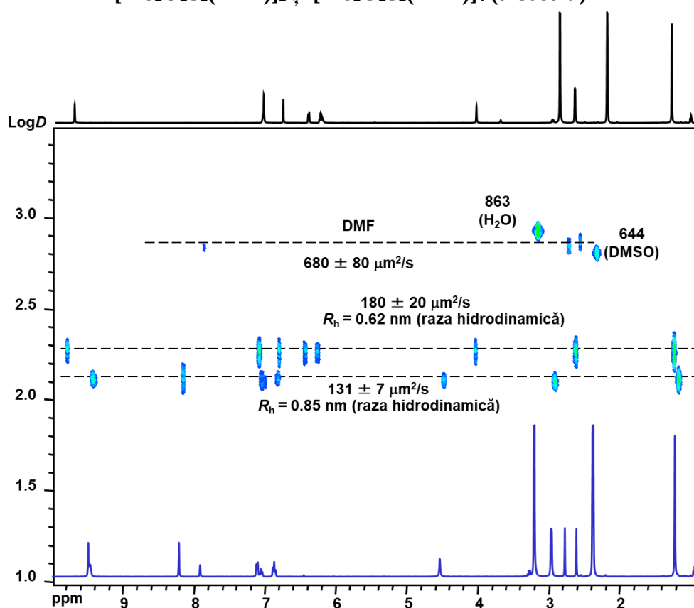
Fig. A9.10 400 MHz ^1\text{H} DOSY RMN ( \text{DMSO-d}_6 ) spectru al ligandului \text{H}_2\text{L}^{19} (negru) și al [\text{Mo}_2\text{O}_2\text{S}_2(\text{L}^{19})]_2 (albastru)
