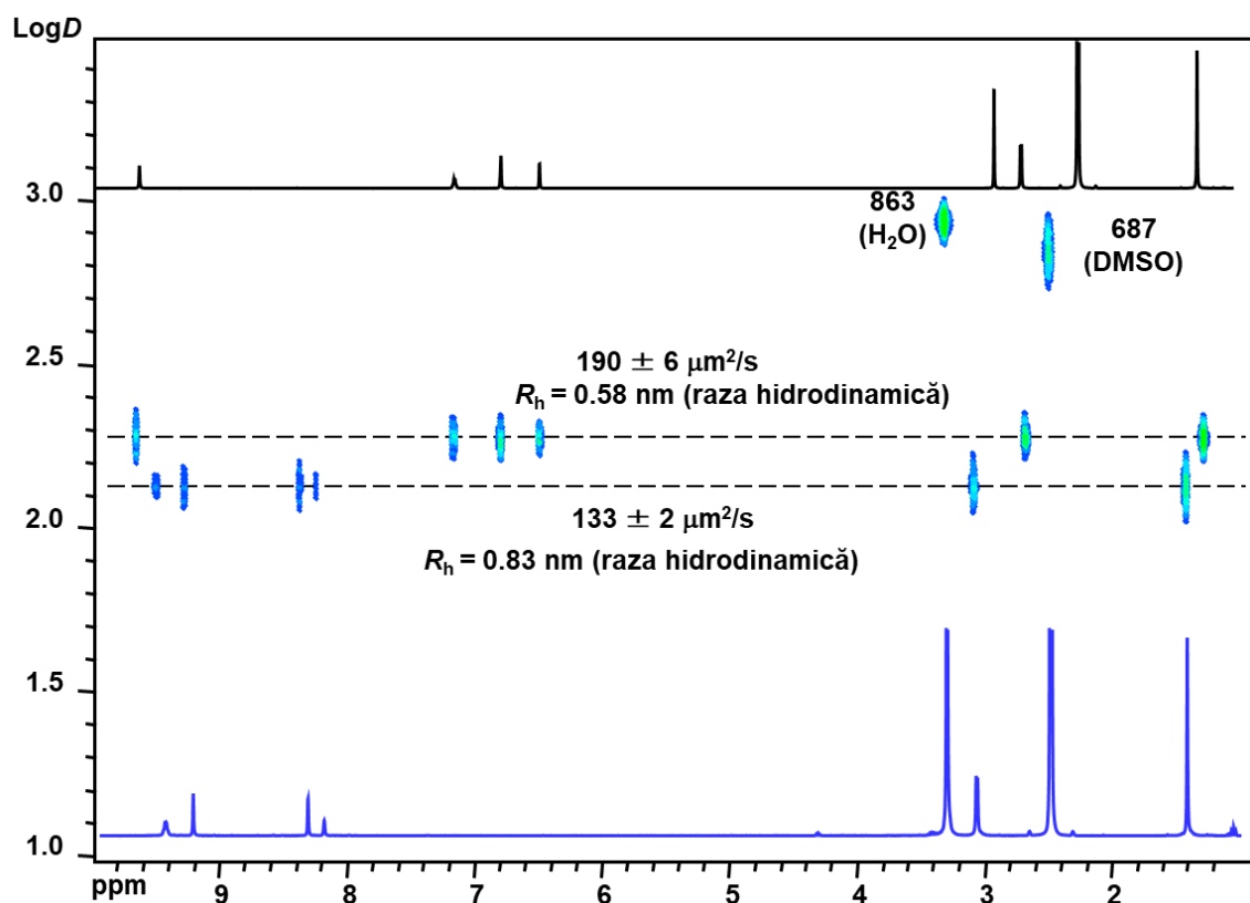
Fig. A9.5 400 MHz ^1\text{H} DOSY RMN (DMSO- \text{d}_6 ) spectru al ligandului \text{H}_2\text{L}^{12} (negru) și al [\text{Mo}_2\text{O}_2\text{S}_2(\text{L}^{12})]_2 (albastru)
