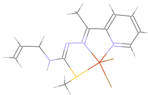
[Cu(HL na )Br 2 ] CCDC 2046083
