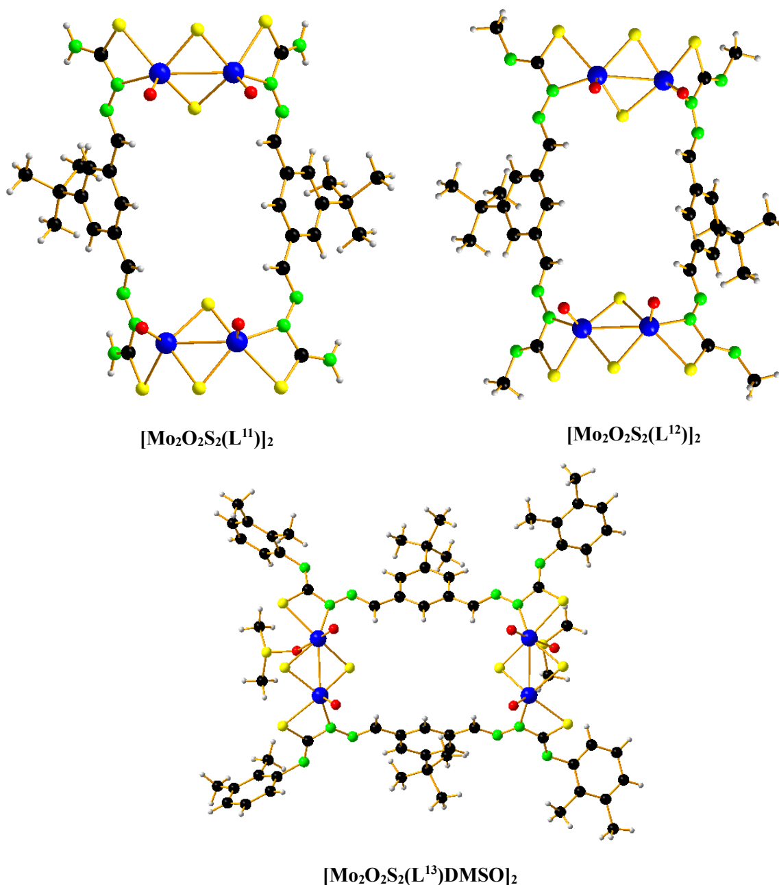
Fig. 4.5. Structurile moleculare ale compușilor cu liganzi rigizi: [\text{Mo}_2\text{O}_2\text{S}_2(\text{L}^{11})]_2 , [\text{Mo}_2\text{O}_2\text{S}_2(\text{L}^{12})]_2 și [\text{Mo}_2\text{O}_2\text{S}_2(\text{L}^{13})\text{DMSO}]_2
