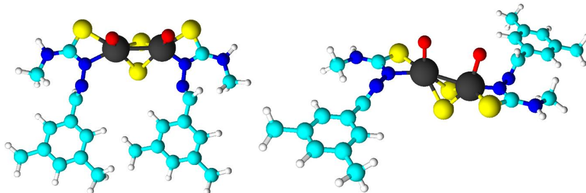
Fig. 3.7. Structura probabilă a complexului ( cis - sau trans -)[Mo 2 O 2 S 2 (L 1 ) 2 ]
