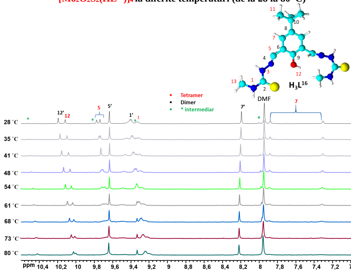
Fig. A8.10 400 MHz ^1\text{H} RMN (DMSO- \text{d}_6 ) spectru al complexului [\text{Mo}_2\text{O}_2\text{S}_2(\text{HL}^{16})]_2 și [\text{Mo}_2\text{O}_2\text{S}_2(\text{HL}^{16})]_4 la diferite temperaturi (de la 28 la 80 °C)
