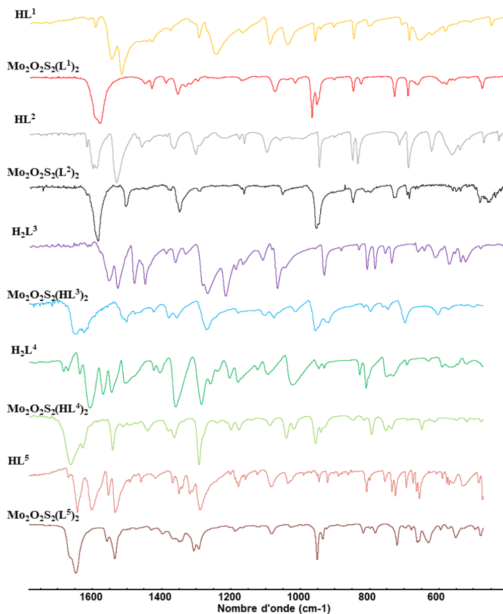
Fig. A1.1 Spectrele infraroșu ale mono-tiosemicarbazonelor și compușilor în baza acestor liganzi [Mo_2O_2S_2(H_nL^{1-5})_2] , n = 0, 1
