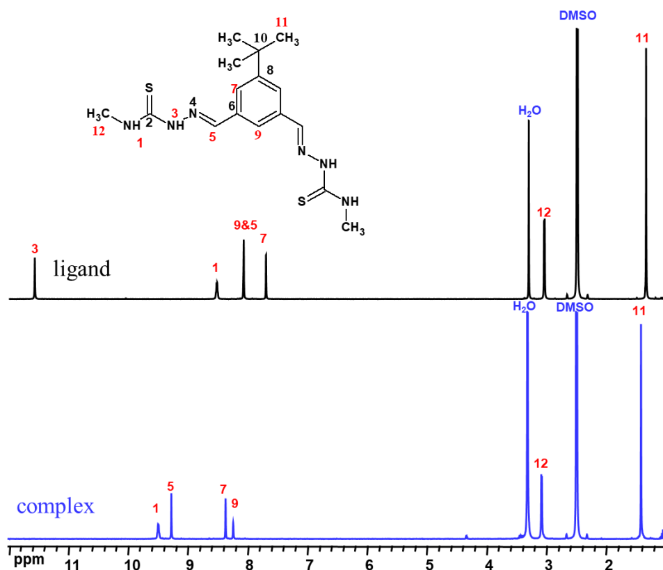
Fig. A8.5 400 MHz ^1H RMN (DMSO- d_6 ) spectru al ligandului H_2L^{12} (negru) și al [Mo_2O_2S_2(L^{12})]_2 (albastru)
