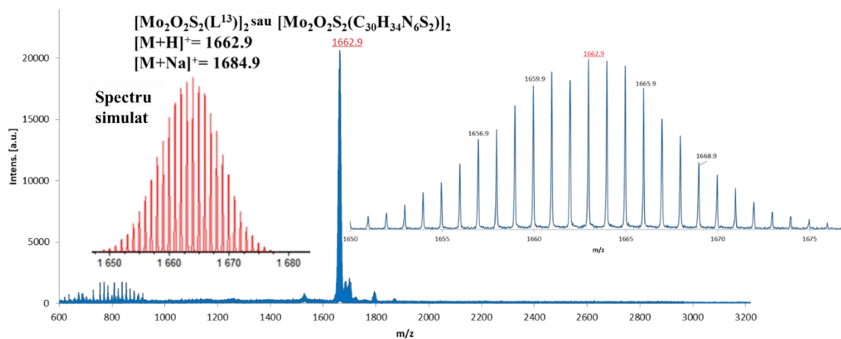
Fig. A6.6 Spectru de masă MALDI-TOF al compusului [\text{Mo}_2\text{O}_2\text{S}_2(\text{L}^{13})]_2
