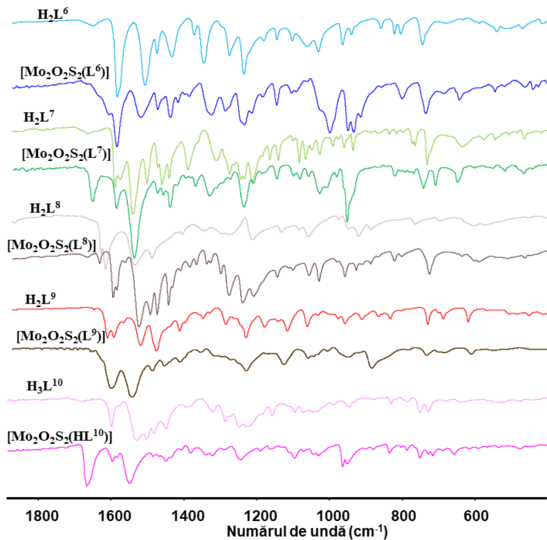
Fig. A5.1 Spectrele infraroșu ale bis-tiosemicarbazonelor flexibile și compușilor în baza Mo V
