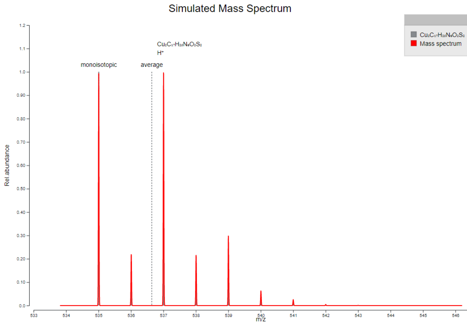
Fig. A6.25 Spectrul de masă simulat al compusului [\text{Cu}_2(\text{HL}^{16})\text{OCH}_3]^+\text{ClO}_4^- prin Prot pi
