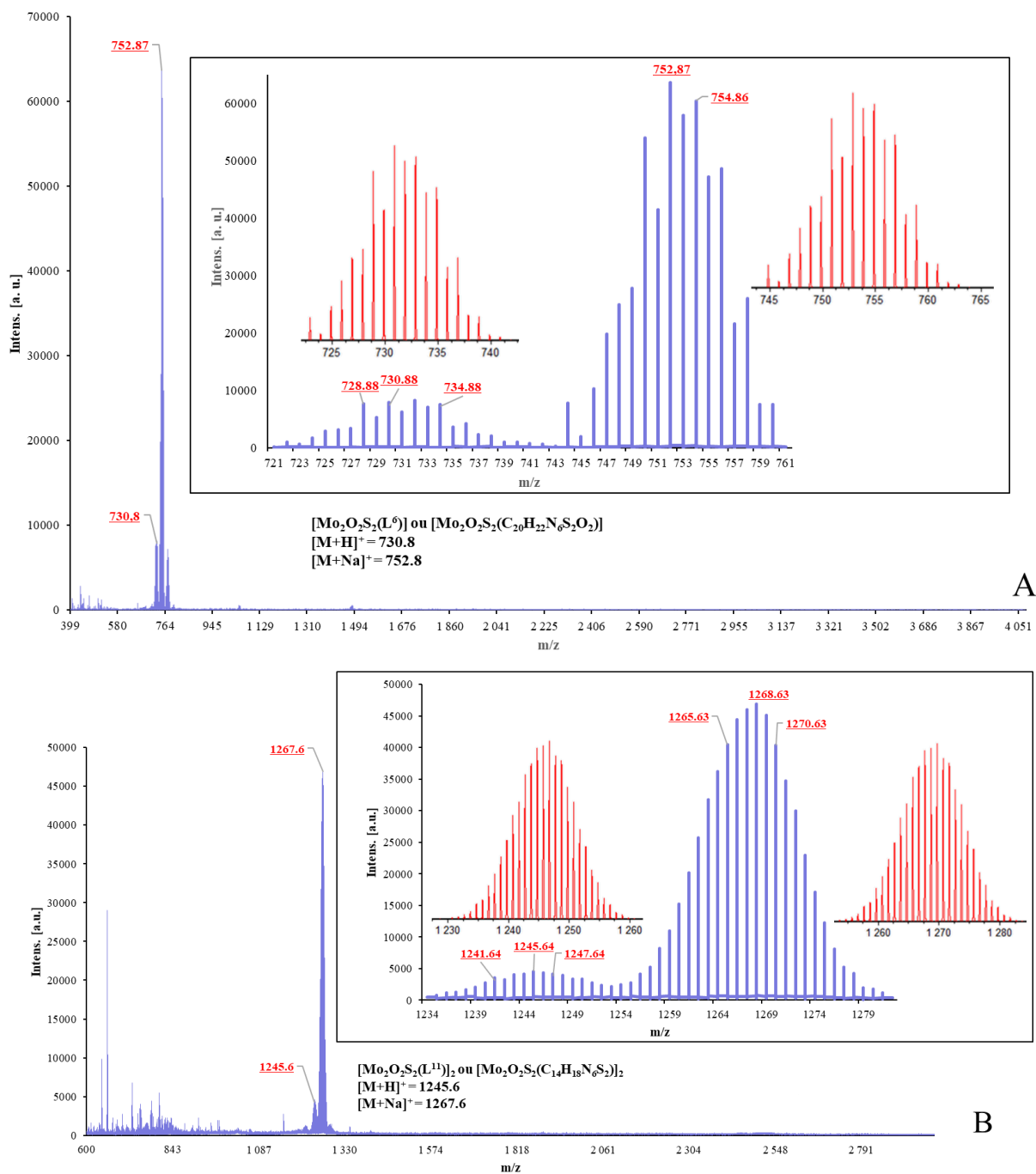
Fig. 4.3. Spectrul de masă MALDI-TOF al compusului [Mo_2O_2S_2(L^6)] (A) și [Mo_2O_2S_2(L^{11})]_2 (B). Spectrele roșii sunt simulate de IsoPro3.
