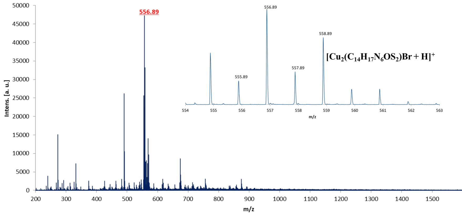
Fig. A6.12 Spectru de masă MALDI-TOF al compusului [\text{Cu}_2(\text{L}^{15})\text{Br}]
