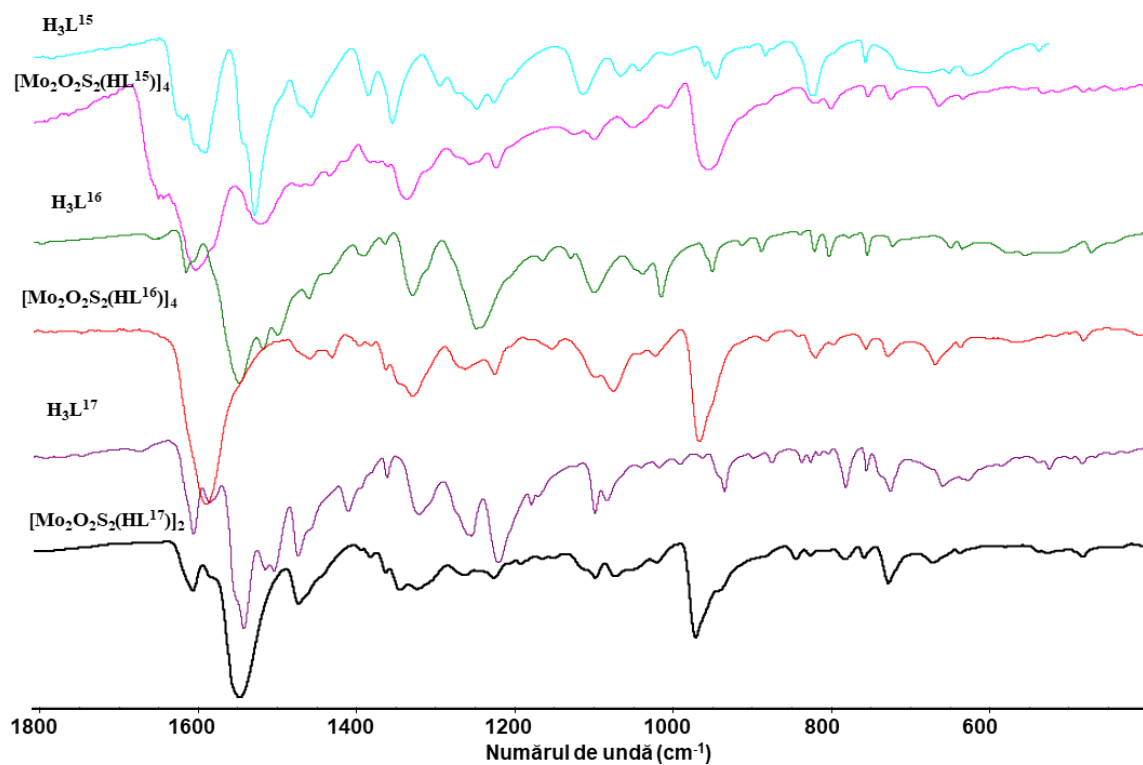
Fig. A5.3 Spectrele infraroșu ale fenol bis-tiosemicarbazonelor și compușilor în baza Mo V
