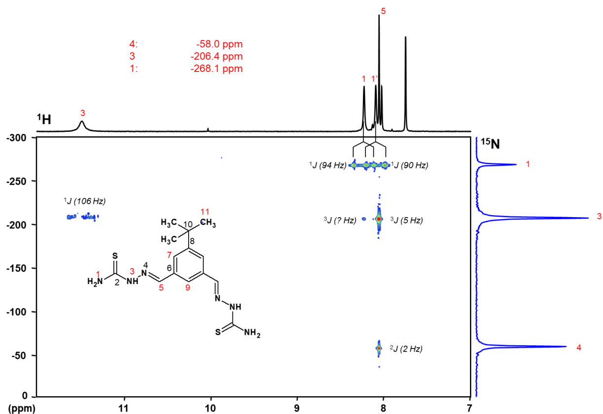
Fig. 4.13. Spectrul RMN 400 MHz ^1\text{H}\{^{15}\text{N}\} HMBC al ligandului \text{H}_2\text{L}^{11} în \text{DMSO-d}_6
