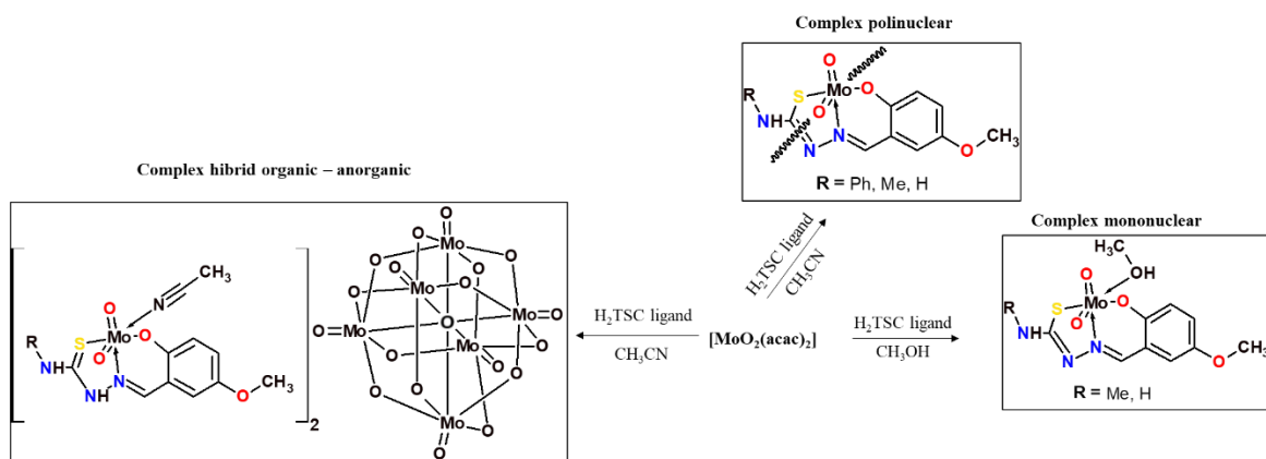
Fig. 1.13. Metoda de sinteză a compușilor polinucleari, mononucleari ai molibdenului (VI) și a complexelor hibridi organici – anorganici cu tiosemicarbazone [49]
