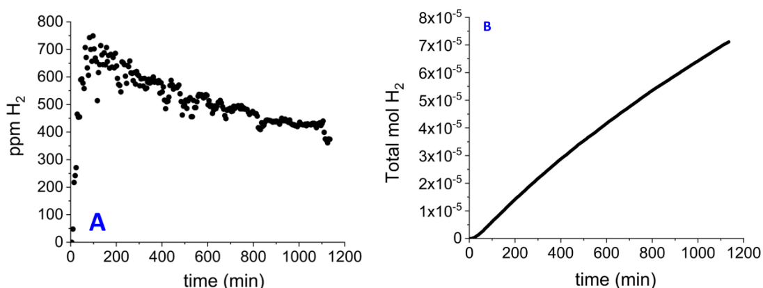
Fig. R. 1. Cantitatea de hidrogen (în ppm – A și mol – B) produsă timp de 20 ore la \text{pH} = 1 și la un potențial constant de -0.6 \text{ V} (Complexul [\text{Mo}_2\text{O}_2\text{S}_2(\text{L}^6)] a fost depus pe un electrod din carbon cu nafion)
