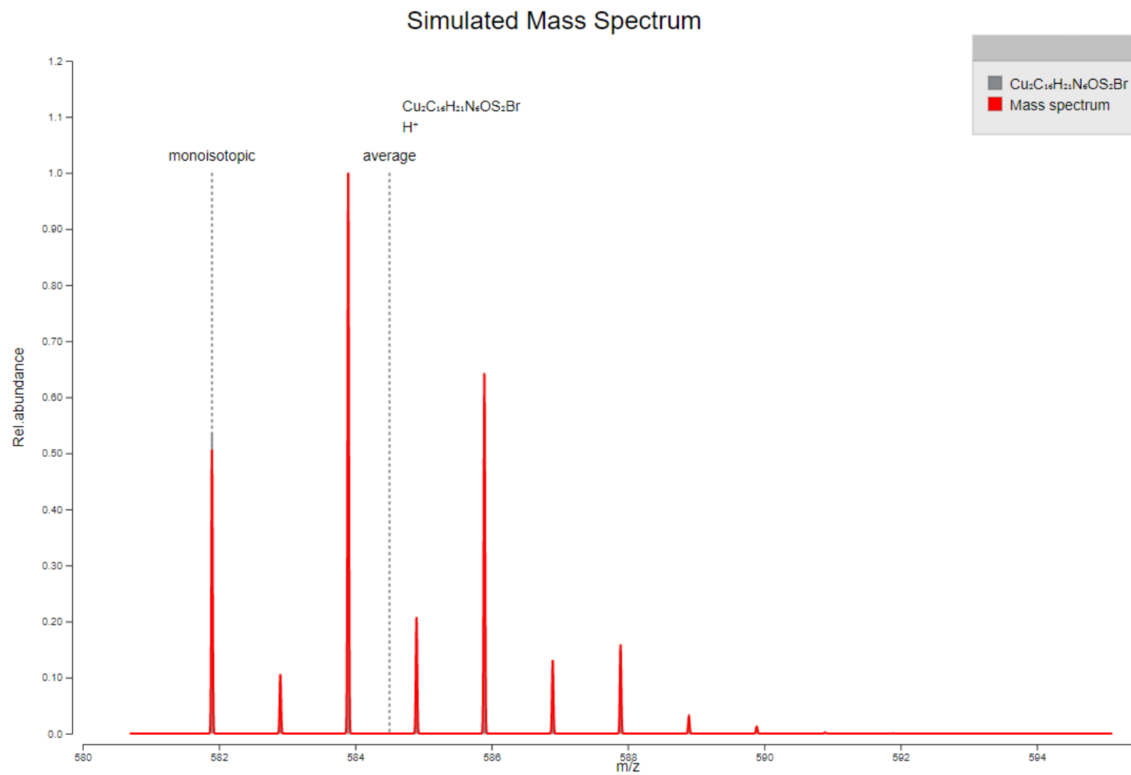
Fig. A6.19 Spectrul de masă simulat al compusului [\text{Cu}_2(\text{L}^{16})\text{Br}] prin Prot pi
