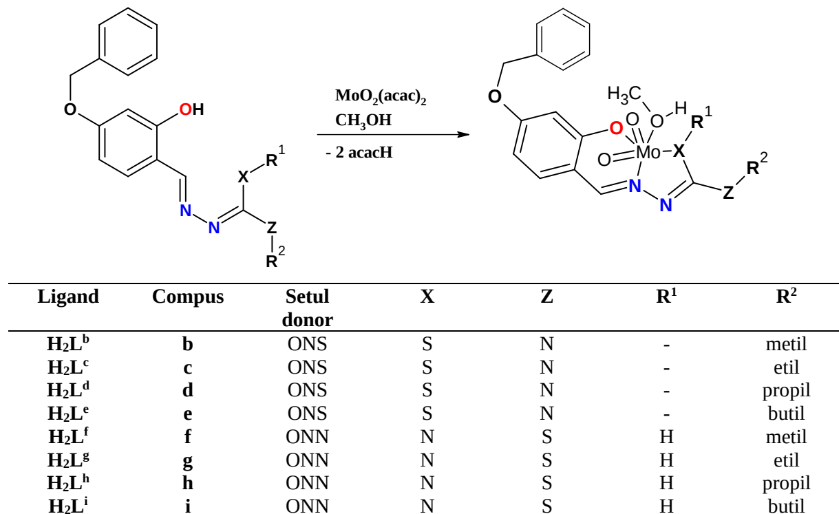
Fig. 1.4. Sinteza compușilor b-i în baza Mo VI [13]
