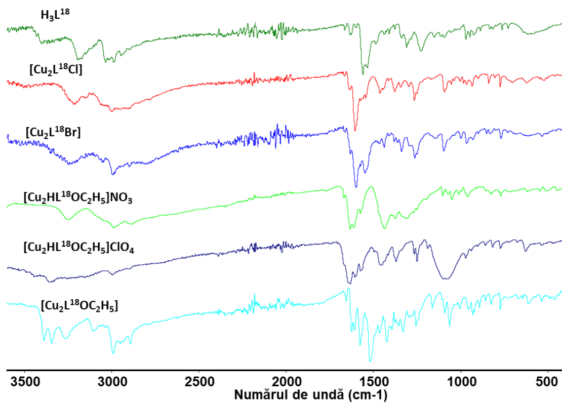
Fig. A5.6 Spectrele IR ale fenol bis-tiosemicarbazonei H 3 L 18 și compușilor de Cu II
