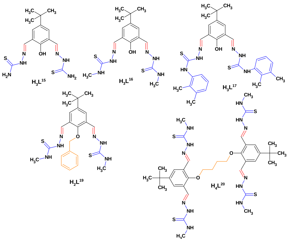
Fig. 4.15. Structurile chimice ale tiosemicarbazonelor \text{H}_3\text{L}^{15-17} , \text{H}_2\text{L}^{19} și \text{H}_4\text{L}^{20}
