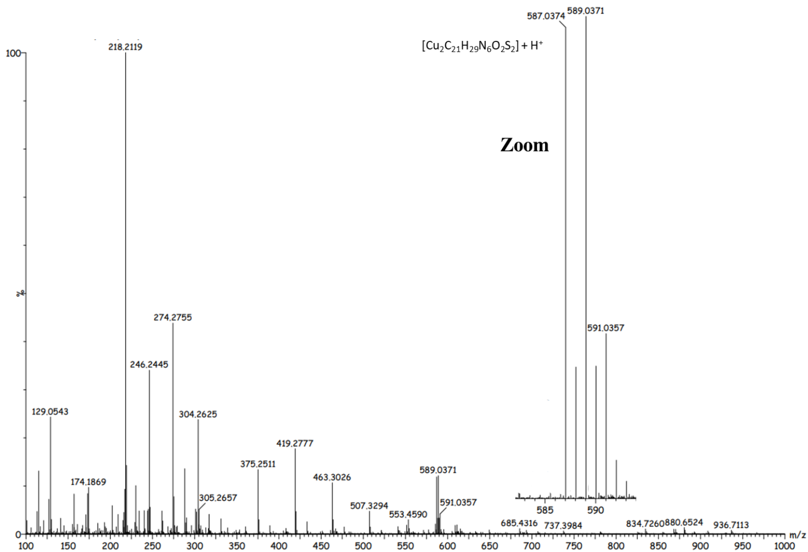
Fig. A6.26 Spectru de masă ESI-MS al compusului \text{Cu}_2(\text{L}^{18})\text{Cl}
