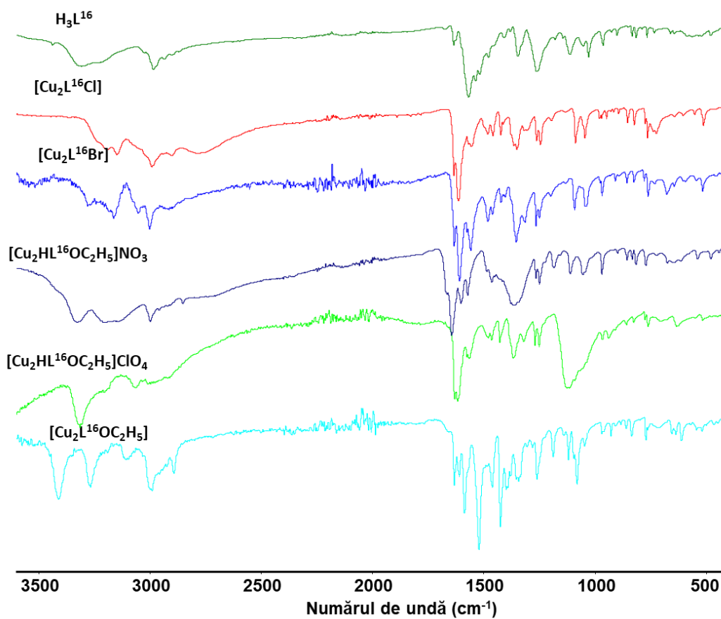
Fig. A5.5 Spectrele IR ale fenol bis-tiosemicarbazonei H_3L^{16} și compușilor de Cu^{II}
