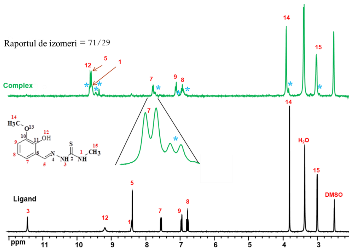
Fig. 3.9. 300 MHz ^1\text{H} RMN ( \text{DMSO-d}_6 ) spectru al ligandului \text{H}_2\text{L}^3 (negru) și complexului [\text{Mo}_2\text{O}_2\text{S}_2(\text{HL}^3)_2] (verde) (Pentru complex, atribuirile în roșu corespund izomerului de 71%, în timp ce atribuirile în * corespund izomerului de 29%)
