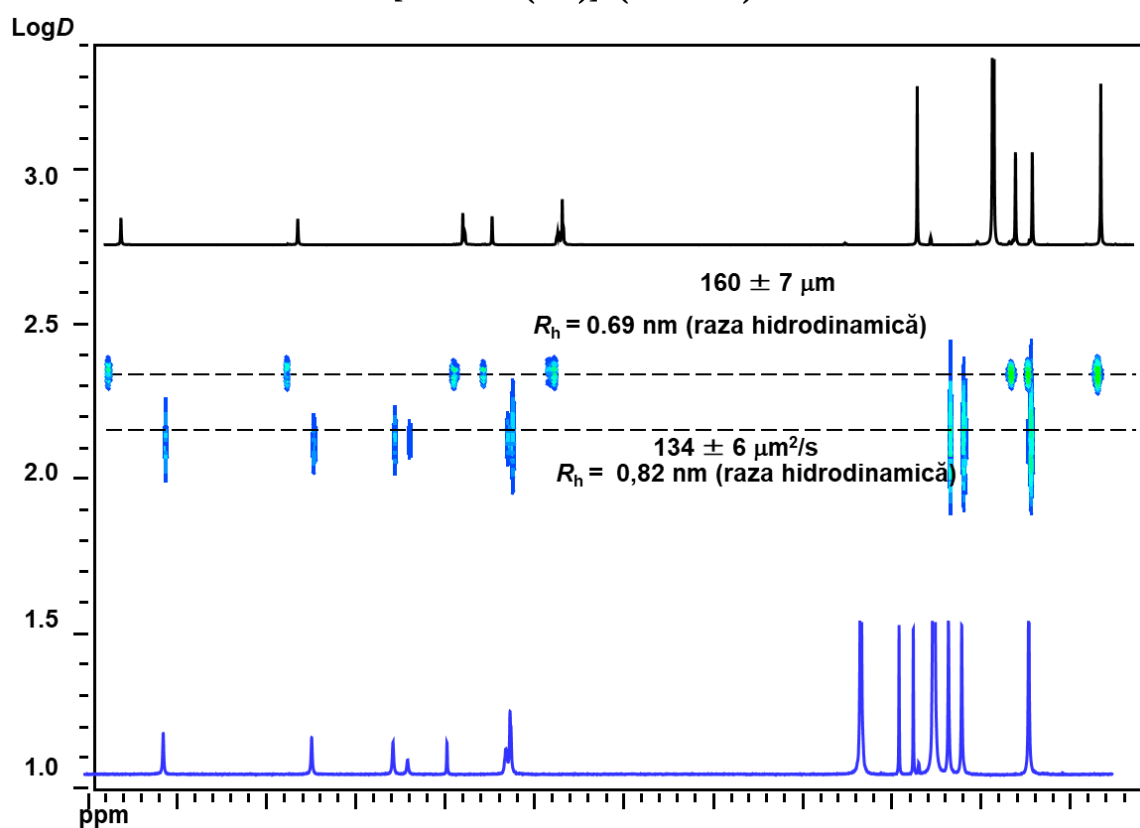
Fig. A9.6 400 MHz ^1\text{H} DOSY RMN (DMSO- \text{d}_6 ) spectru al ligandului \text{H}_2\text{L}^{13} (negru) și al [\text{Mo}_2\text{O}_2\text{S}_2(\text{L}^{13})]_2 (albastru)
