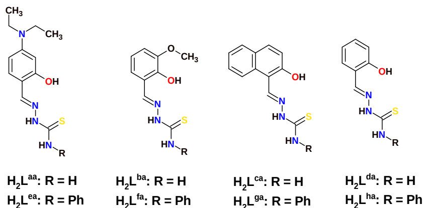
Fig. 1.11. Structura tiosemicarbazonelor H_2L^{aa-ha} [45]
