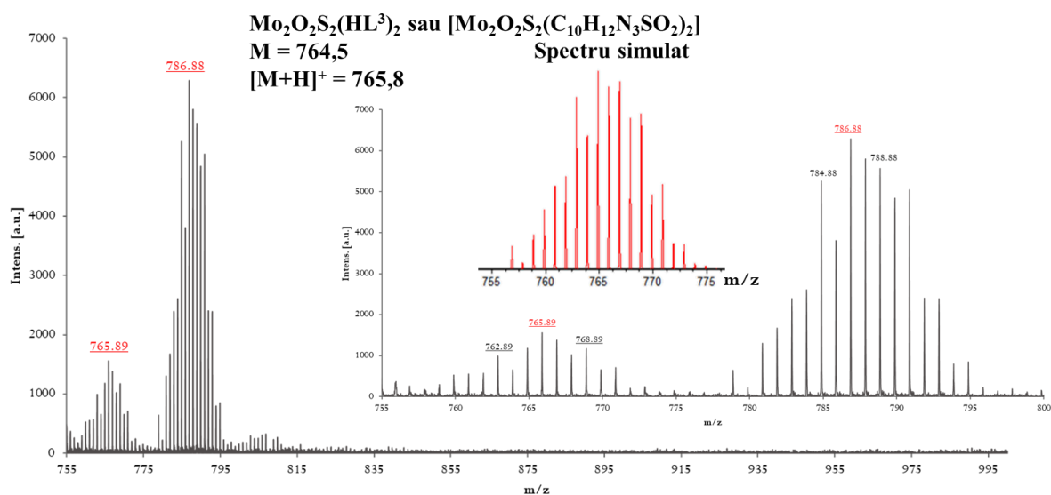
Fig. A2.7 Spectru de masă MALDI-TOF al compusului [\text{Mo}_2\text{O}_2\text{S}_2(\text{HL}^3)_2]
