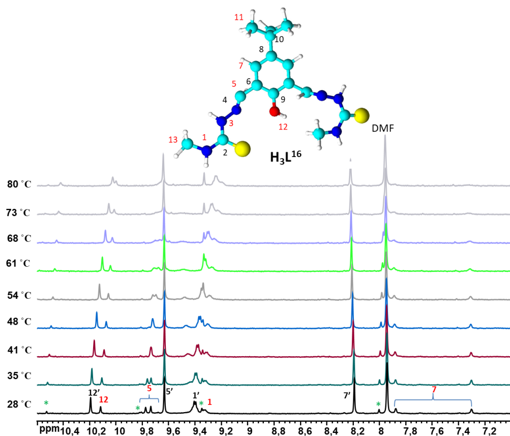
Fig. A8.12 400 MHz ^1\text{H} RMN (DMSO- d_6 ) spectru al complexului [\text{Mo}_2\text{O}_2\text{S}_2(\text{HL}^{16})]_2 și [\text{Mo}_2\text{O}_2\text{S}_2(\text{HL}^{16})]_4 la diferite temperaturi (de la 80 la 28 °C)
