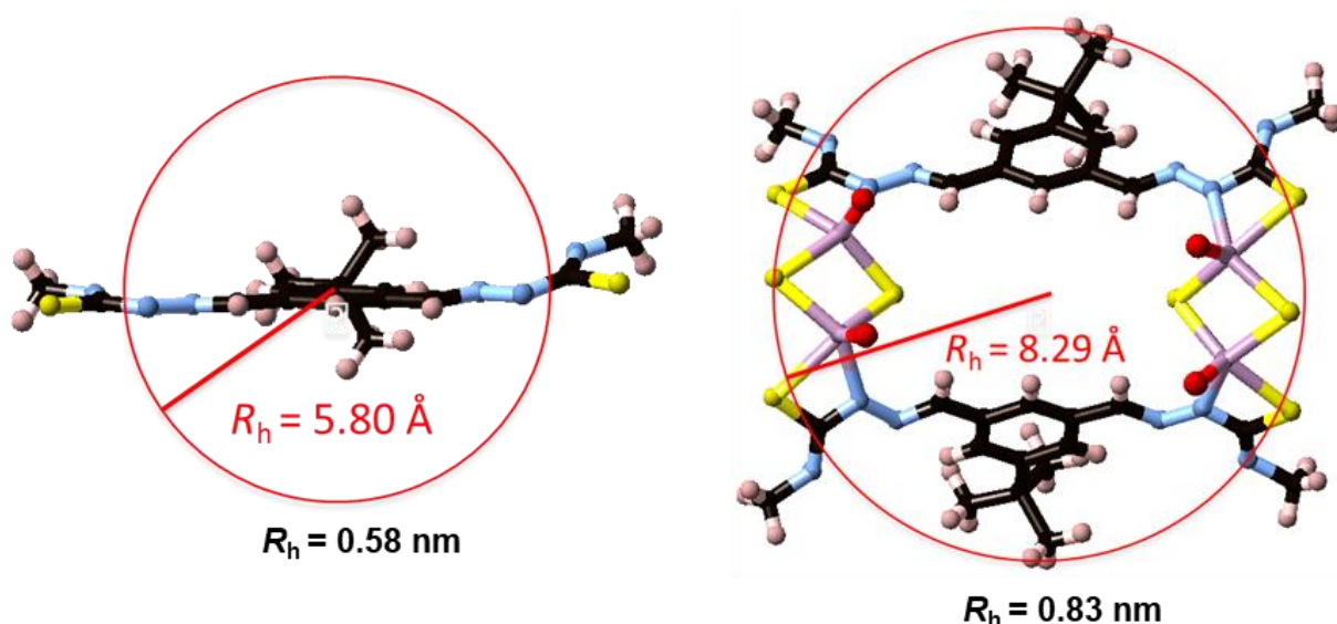
Fig. 4.10. Valorile razelor hidrodinamice conform analizei cu raze X (roșie) și DOSY (negru) ale \text{H}_2\text{L}^{12} și [\text{Mo}_2\text{O}_2\text{S}_2(\text{L}^{12})]_2
