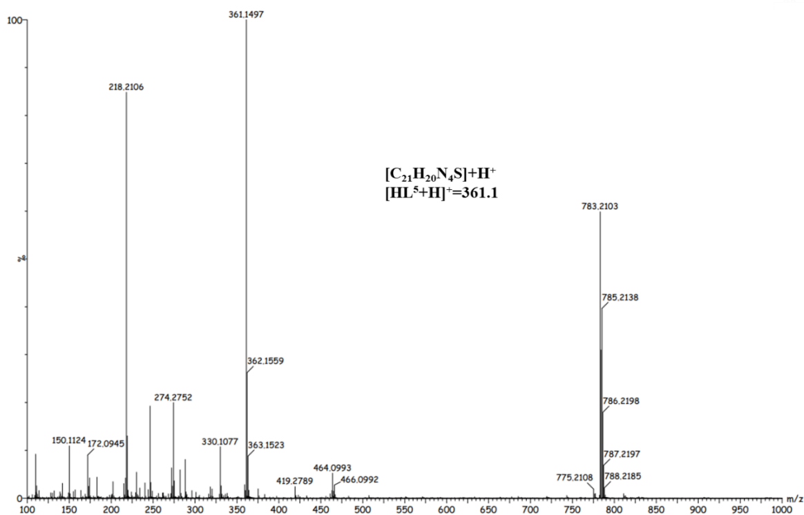
Fig. A2.5 Spectru de masă ESI-MS al mono-tiosemicarbazonei HL^5
