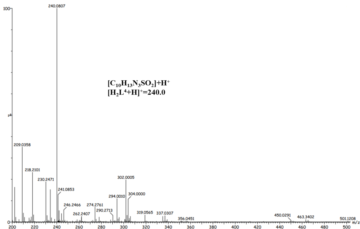
Fig. A2.4 Spectru de masă ESI-MS al mono-tiosemicarbazonei H_2L^4
