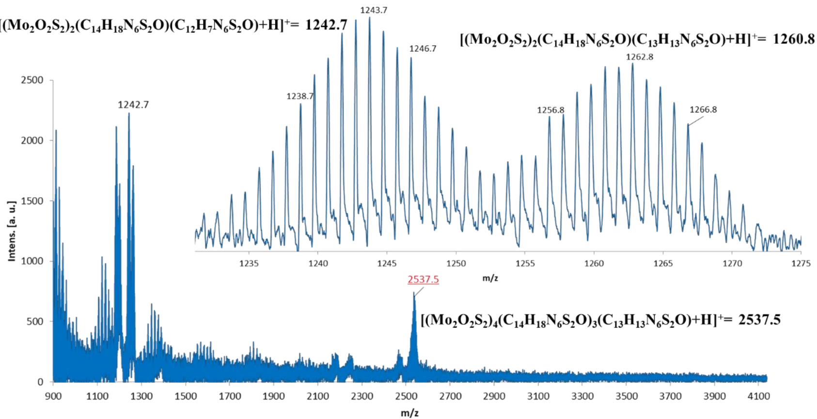
Fig. A6.9 Spectru de masă MALDI-TOF al compusului [\text{Mo}_2\text{O}_2\text{S}_2(\text{HL}^{15})]_2 și \text{Mo}_2\text{O}_2\text{S}_2(\text{HL}^{15})_4
