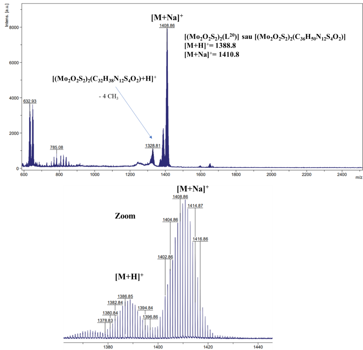
Fig. A6.11 Spectru de masă MALDI-TOF al compusului [(\text{Mo}_2\text{O}_2\text{S}_2)_2\text{L}^{20}]
