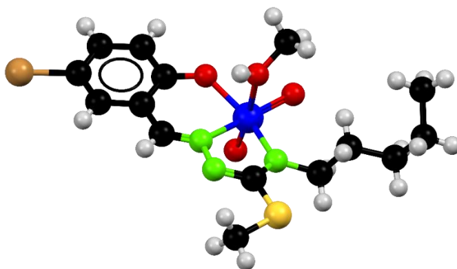
Fig. 1.6. Structura cristalină a compusului (metanol)-(metil N'-(5-bromo-2-oxibenziliden)-N-pentilcarbamohidrazonotioato)-dioxo-molibdenum(VI) (ONN) CCDC 1497812 [40]
