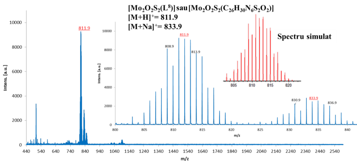
Fig. A6.2 Spectru de masă MALDI-TOF al compusului [Mo 2 O 2 S 2 (L 8 )]
