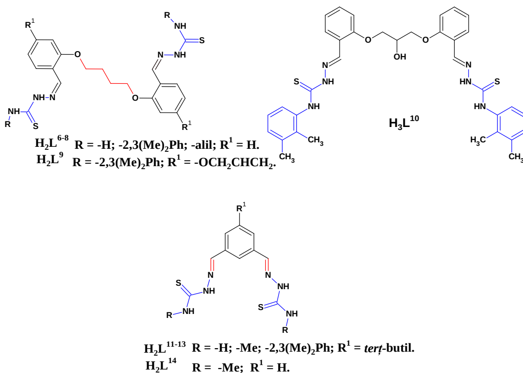
Fig. 4.1. Structurile bis-tiosemicarbazonei flexibile ( \text{H}_2\text{L}^{6-9} și \text{H}_3\text{L}^{10} ) și rigide ( \text{H}_2\text{L}^{11-14} ) sintetizate
