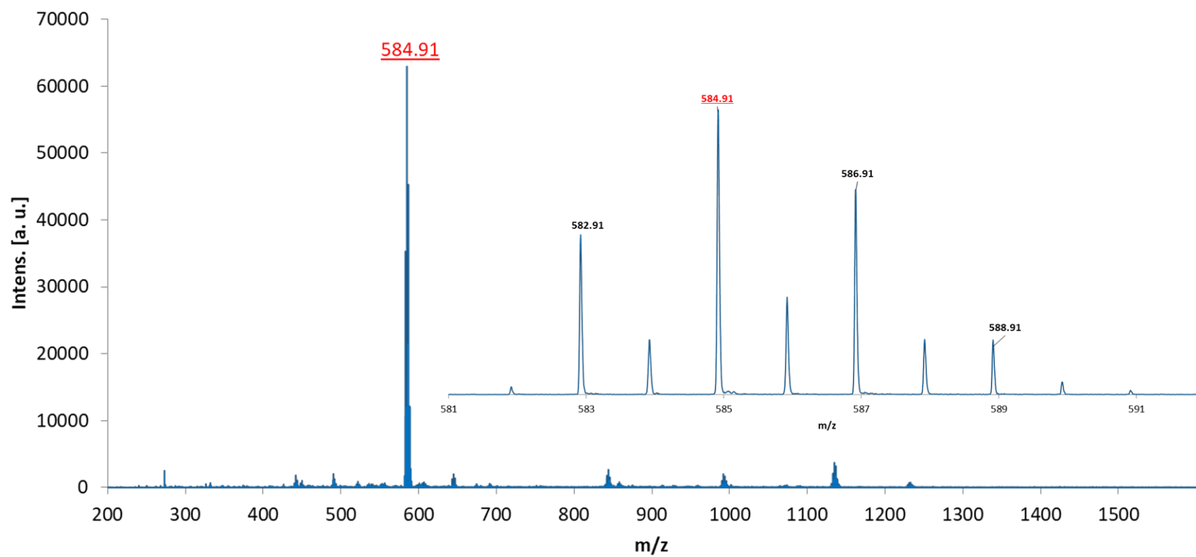
Fig. A6.18 Spectru de masă MALDI-TOF al compusului [\text{Cu}_2(\text{L}^{16})\text{Br}]
