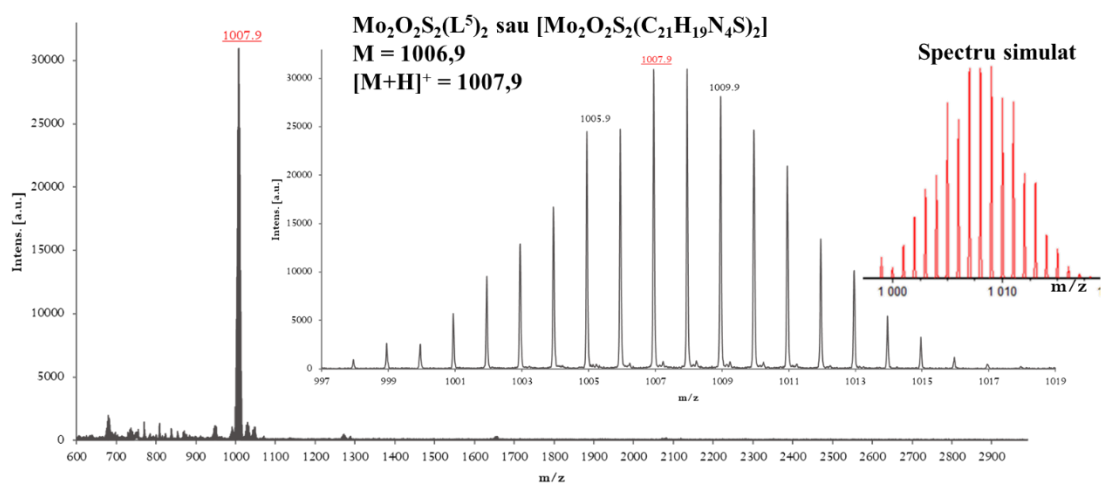
Fig. A2.9 Spectru de masă MALDI-TOF al compusului [\text{Mo}_2\text{O}_2\text{S}_2(\text{L}^5)_2]
