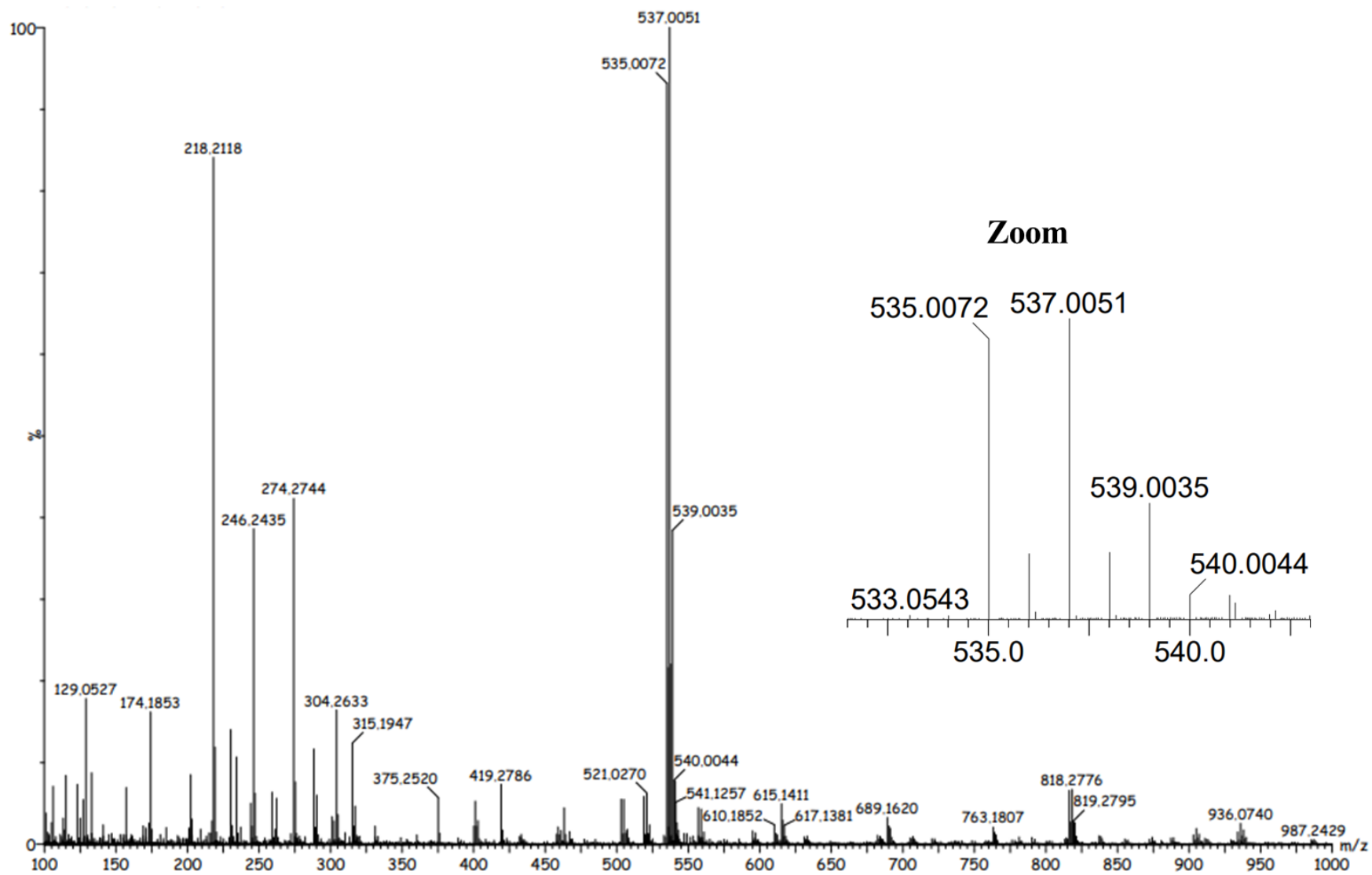
Fig. A6.22 Spectru de masă ESI-MS al compusului \text{Cu}_2\text{L}^{16}\text{Cl}
