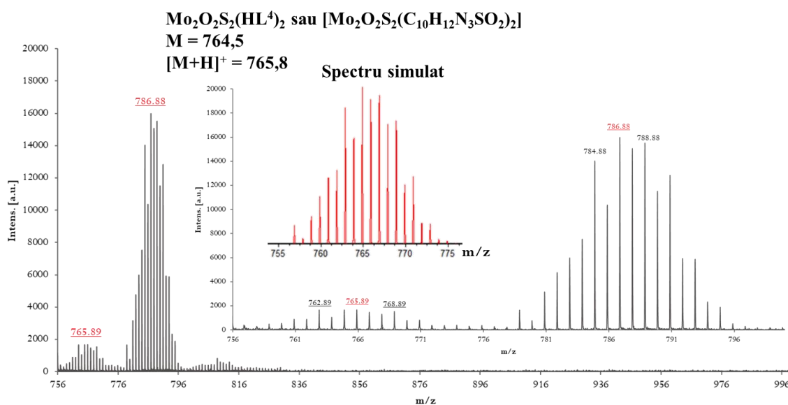
Fig. A2.8 Spectru de masă MALDI-TOF al compusului [\text{Mo}_2\text{O}_2\text{S}_2(\text{HL}^4)_2]
