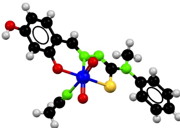
Fig. 1.12. Structura cristalină a compusului [MoO 2 L ia (CH 3 CN)] CCDC 895788 [7]
