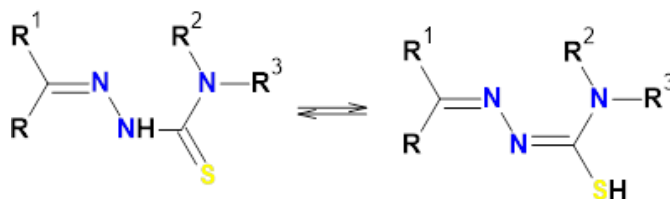
Fig. 1.2. Structura generală a tiosemicarbazonele (tautomeri: tion și tiol)
