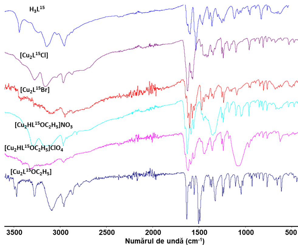
Fig. A5.4 Spectrele IR ale fenol bis-tiosemicarbazonei H_3L^{15} și compușilor de Cu^{II}
