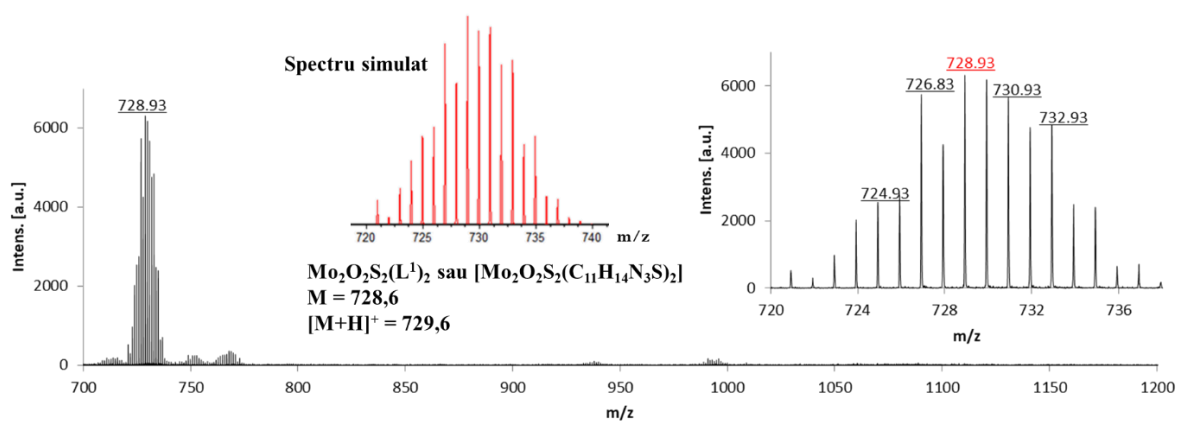
Fig. A2.6 Spectru de masă MALDI-TOF al compusului [Mo_2O_2S_2(L^1)_2]
