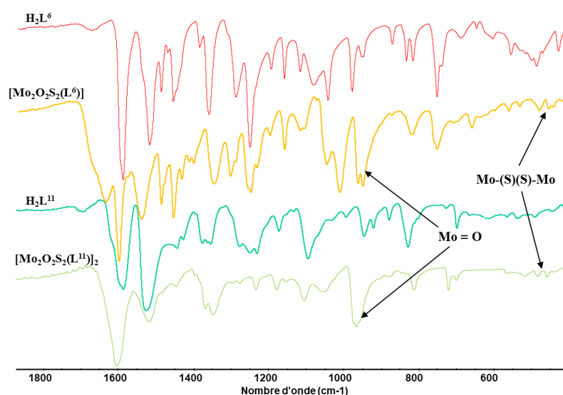
Fig. 4.2. Spectrele IR ale bis-tiosemicarbazonelor \text{H}_2\text{L}^6 , \text{H}_2\text{L}^{11} și compușilor [\text{Mo}_2\text{O}_2\text{S}_2(\text{L}^6)] și [\text{Mo}_2\text{O}_2\text{S}_2(\text{L}^{11})]_2
