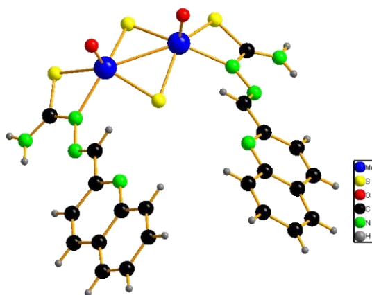
Izomerul cis
