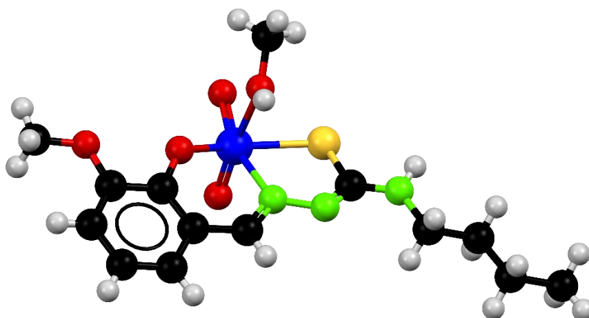
Fig. 1.7. Structura cristalină a compusului k (ONS) CCDC 1540754 [41]
