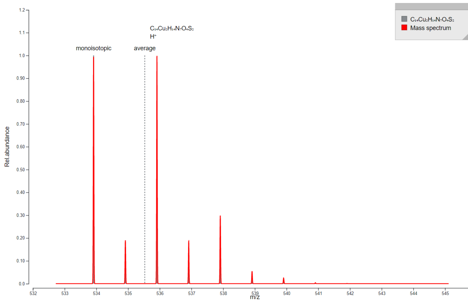
Fig. A6.21 Spectrul de masă simulat al compusului [\text{Cu}_2(\text{HL}^{16})\text{OCH}_3]\text{NO}_3 prin Prot pi
