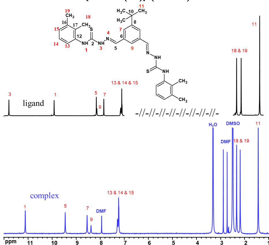
Fig. A8.6 400 MHz ^1H RMN (DMSO- d_6 ) spectru al ligandului H_2L^{13} (negru) și al [Mo_2O_2S_2(L^{13})]_2 (albastru)
