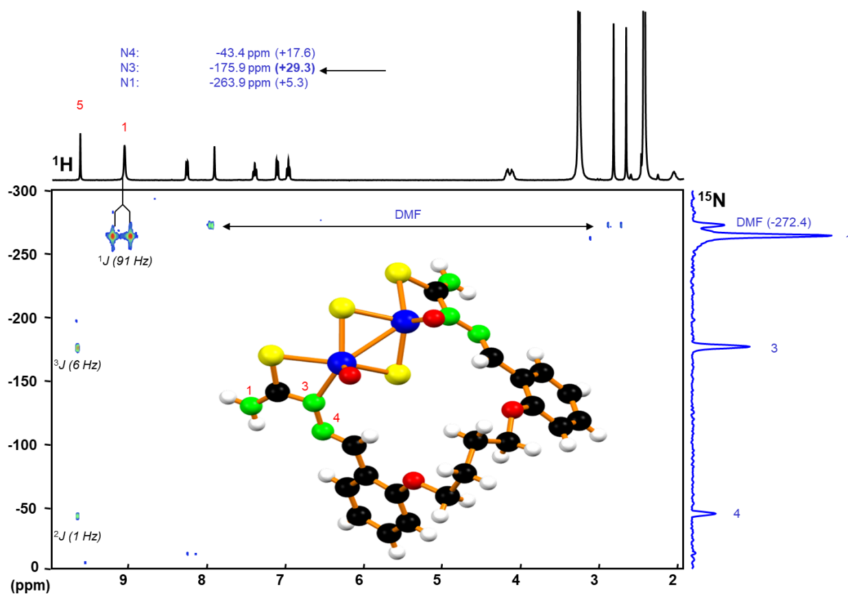
Fig. 4.12. Spectrul RMN 400 MHz ^1\text{H}\{^{15}\text{N}\} HMBC al [\text{Mo}_2\text{O}_2\text{S}_2(\text{L}^6)] în \text{DMSO-d}_6
