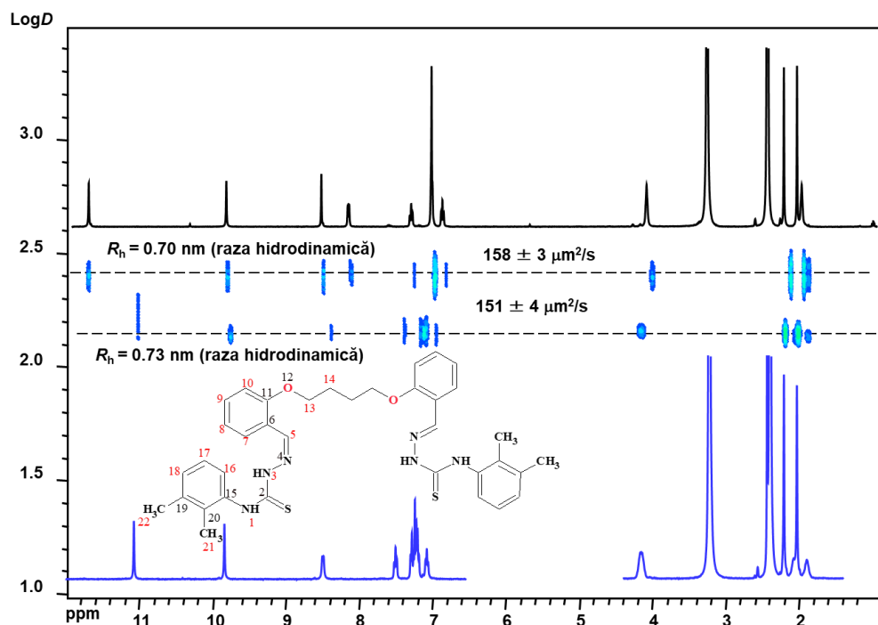
Fig. A9.1 400 MHz ^1\text{H} DOSY RMN ( \text{DMSO-d}_6 ) spectru al ligandului \text{H}_2\text{L}^7 (negru) și al [\text{Mo}_2\text{O}_2\text{S}_2(\text{L}^7)] (albastru)
