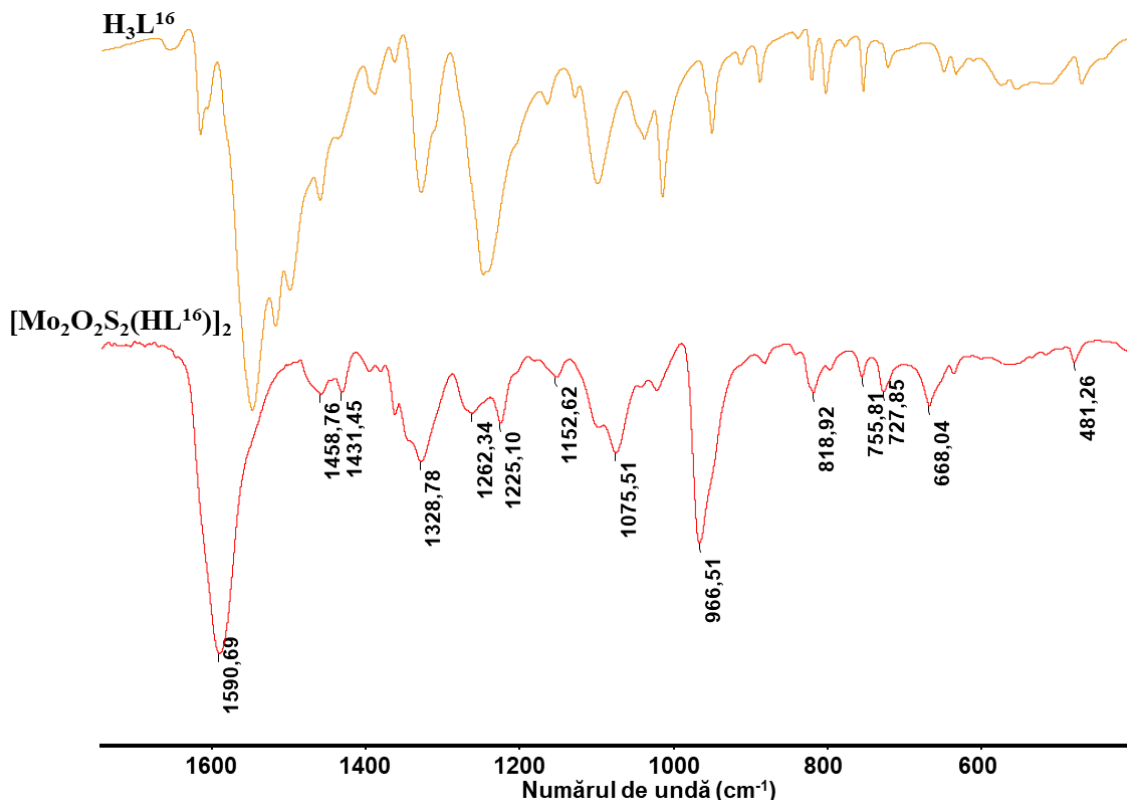
Fig. 4.16. Spectrele IR ale bis-tiosemicarbazonei \text{H}_3\text{L}^{16} și compusului [\text{Mo}_2\text{O}_2\text{S}_2(\text{HL}^{16})]_4
