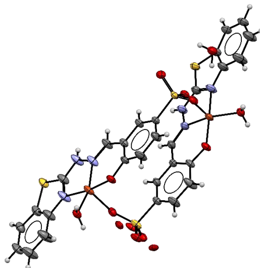
Fig. 1.16. Structura cristalină a complexului [Cu(L cycl )] 2 CCDC 1494080 [55]
