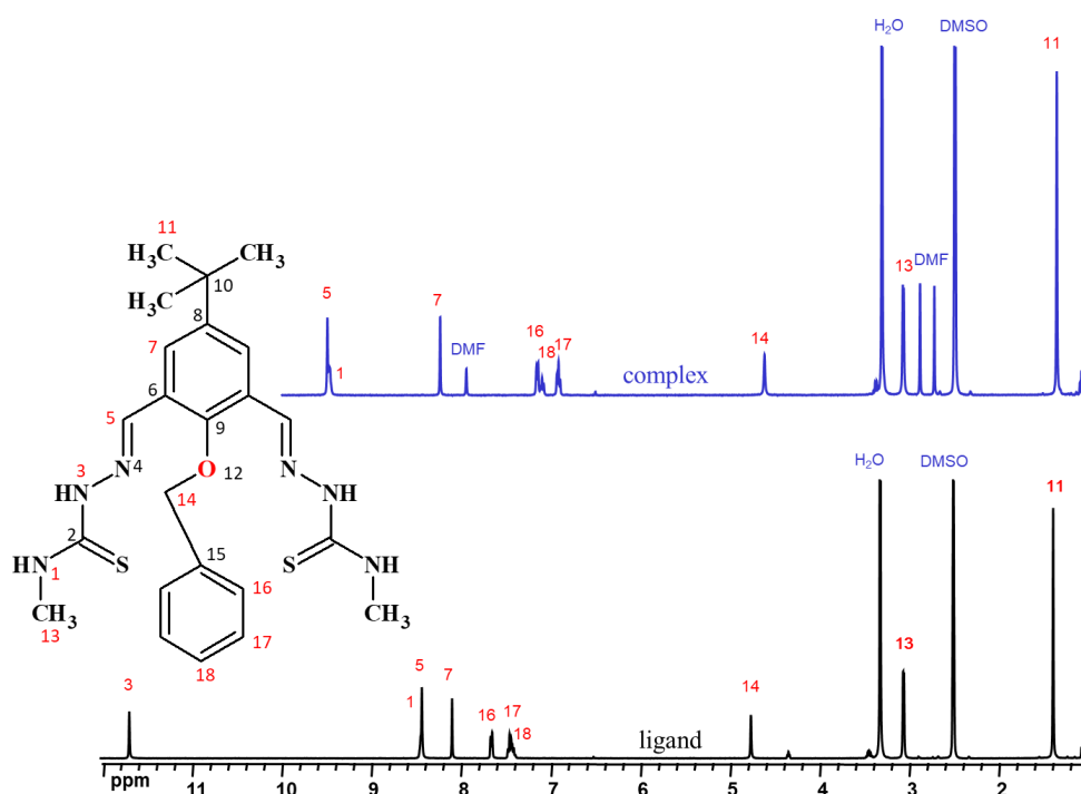
Fig. 4.28. 400 MHz ^1\text{H} RMN ( \text{DMSO-d}_6 ) spectru al ligandului \text{H}_2\text{L}^{19} (negru) și complexului [\text{Mo}_2\text{O}_2\text{S}_2(\text{L}^{19})]_2 (albastru)
