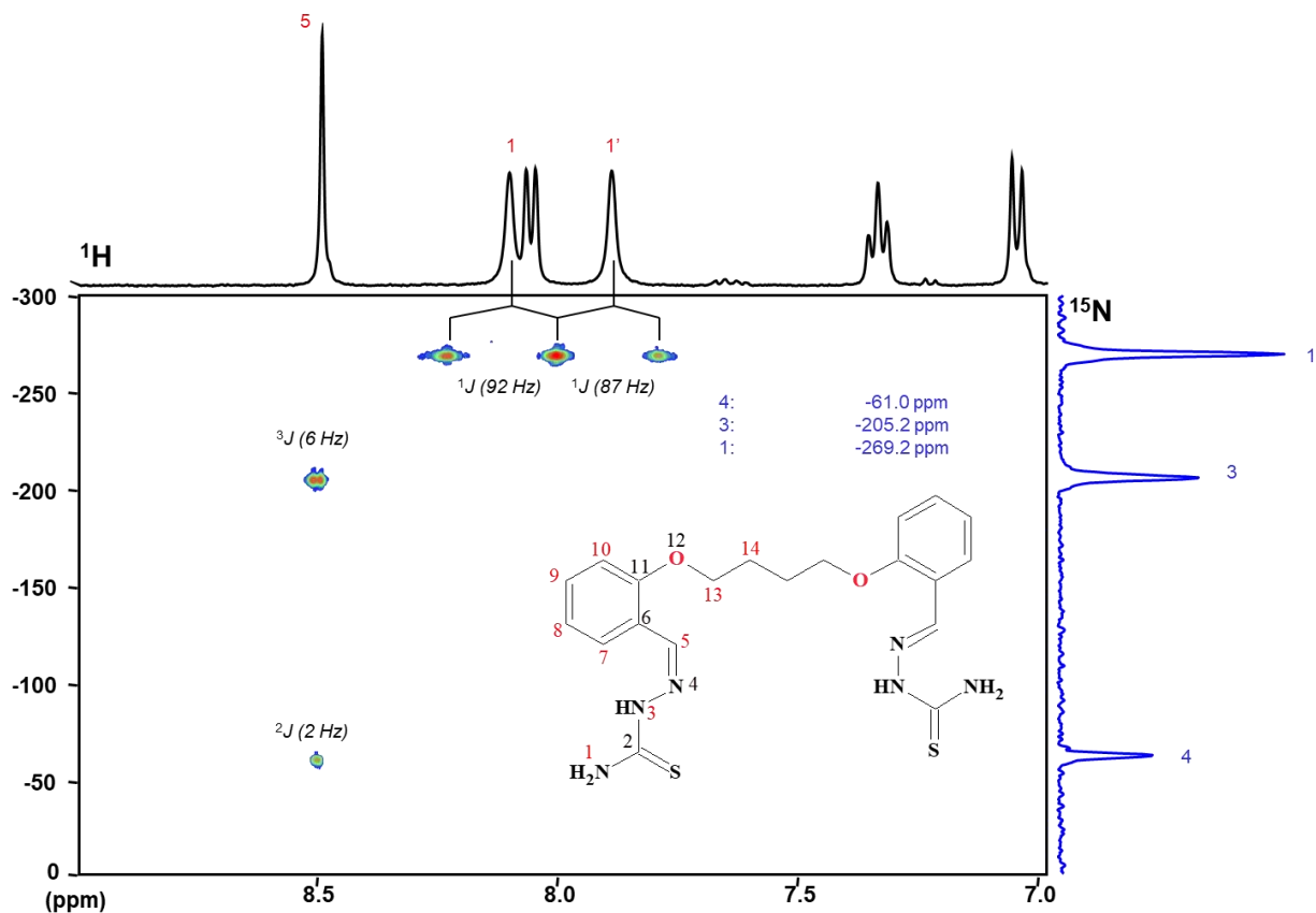
Fig. 4.11. Spectrul RMN 400 MHz ^1\text{H}\{^{15}\text{N}\} HMBC al ligandului H 2 L 6 în DMSO- \text{d}_6
