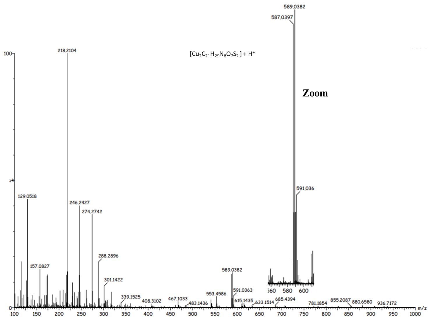
Fig. A6.28 Spectru de masă ESI-MS al compusului [\text{Cu}_2(\text{HL}^{18})\text{OCH}_3]^+\text{NO}_3^-
