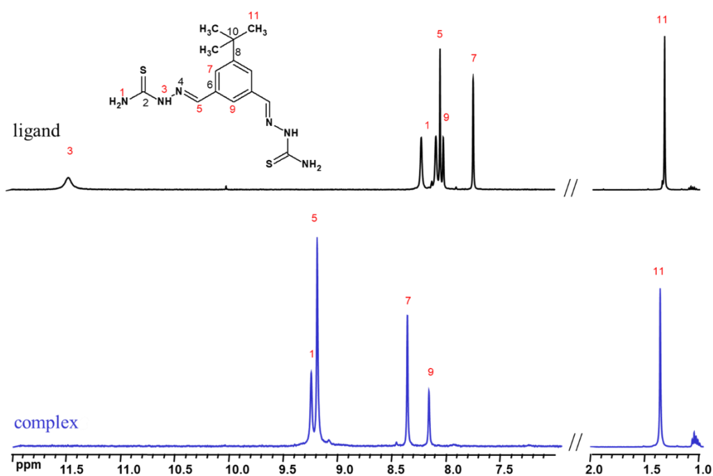
Fig. 4.7. 400 MHz 1 H RMN (DMSO-d 6 ) spectru al ligandului H 2 L 11 (negru) și al [Mo 2 O 2 S 2 (L 11 )] 2 (albastru)
