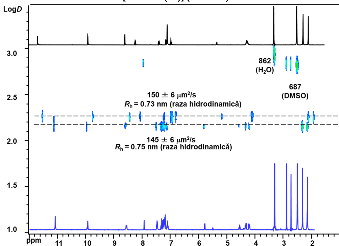
Fig. A9.4 400 MHz ^1\text{H} DOSY RMN (DMSO- d_6 ) spectru al ligandului \text{H}_3\text{L}^{10} (negru) și al [\text{Mo}_2\text{O}_2\text{S}_2(\text{HL}^{10})] (albastru)
