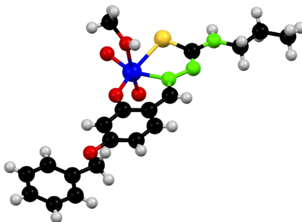
Fig. 1.5. Structura cristalină a complexului d (ONS) CCDC 2081687 [13]
