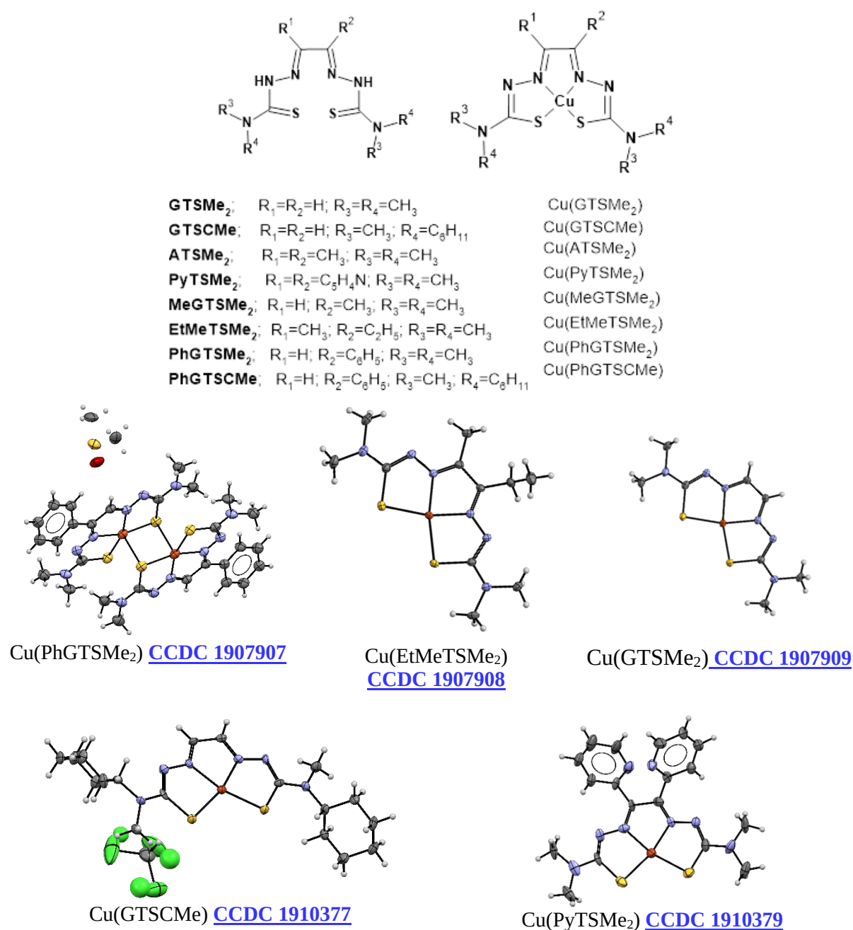
Fig. 1.21. Structura bis-tiosemicarbazonei și compușilor de coordonare [59]
