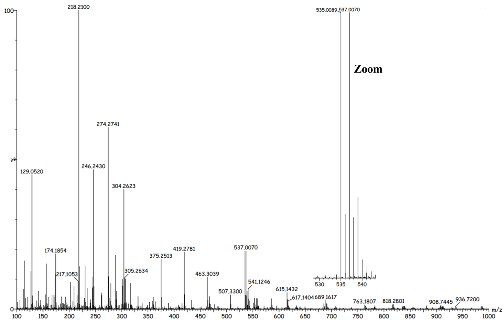
Fig. A6.24 Spectru de masă ESI-MS al compusului [\text{Cu}_2(\text{HL}^{16})\text{OCH}_3]^+\text{ClO}_4^-
