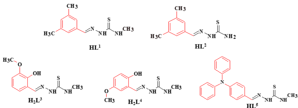
Fig. 2.1. Structurile chimice ale mono-tiosemicarbazonelor HL 1-2,5 și H 2 L 3-4
