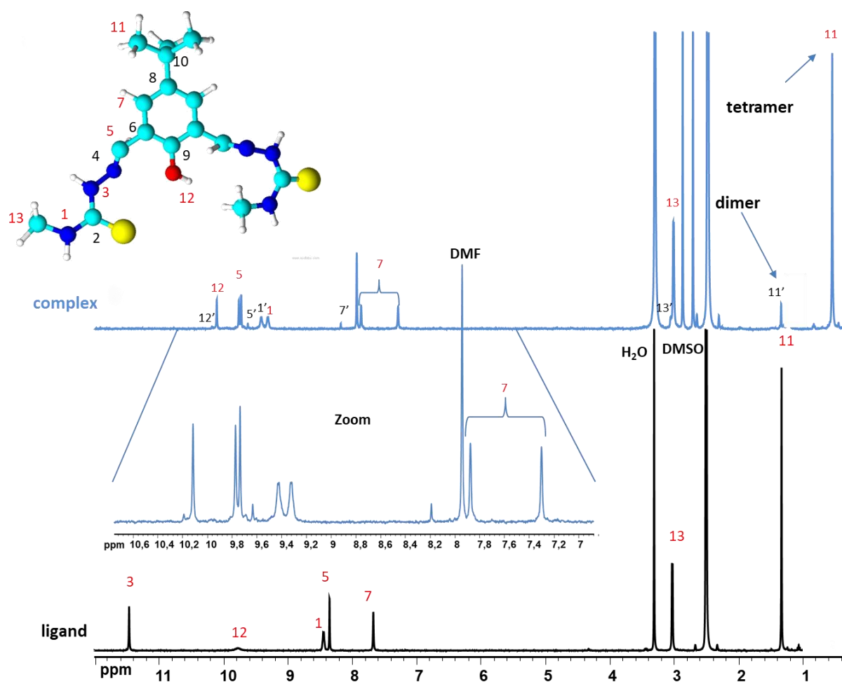
Fig. 4.23. 400 MHz 1 H RMN (DMSO-d 6 ) spectrul ligandului H 3 L 16 (negru) și compusului (albastru, pentru complex, atribuirile în roșu corespund speciei tetramer, în timp ce în negru corespund speciei dimer)
