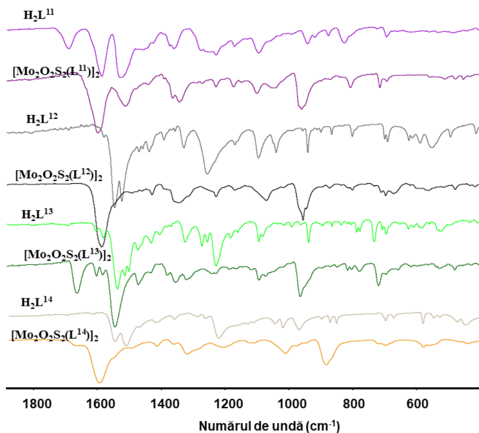
Fig. A5.2 Spectrele infraroșu ale bis-tiosemicarbazonelor rigide și compușilor în baza Mo V
