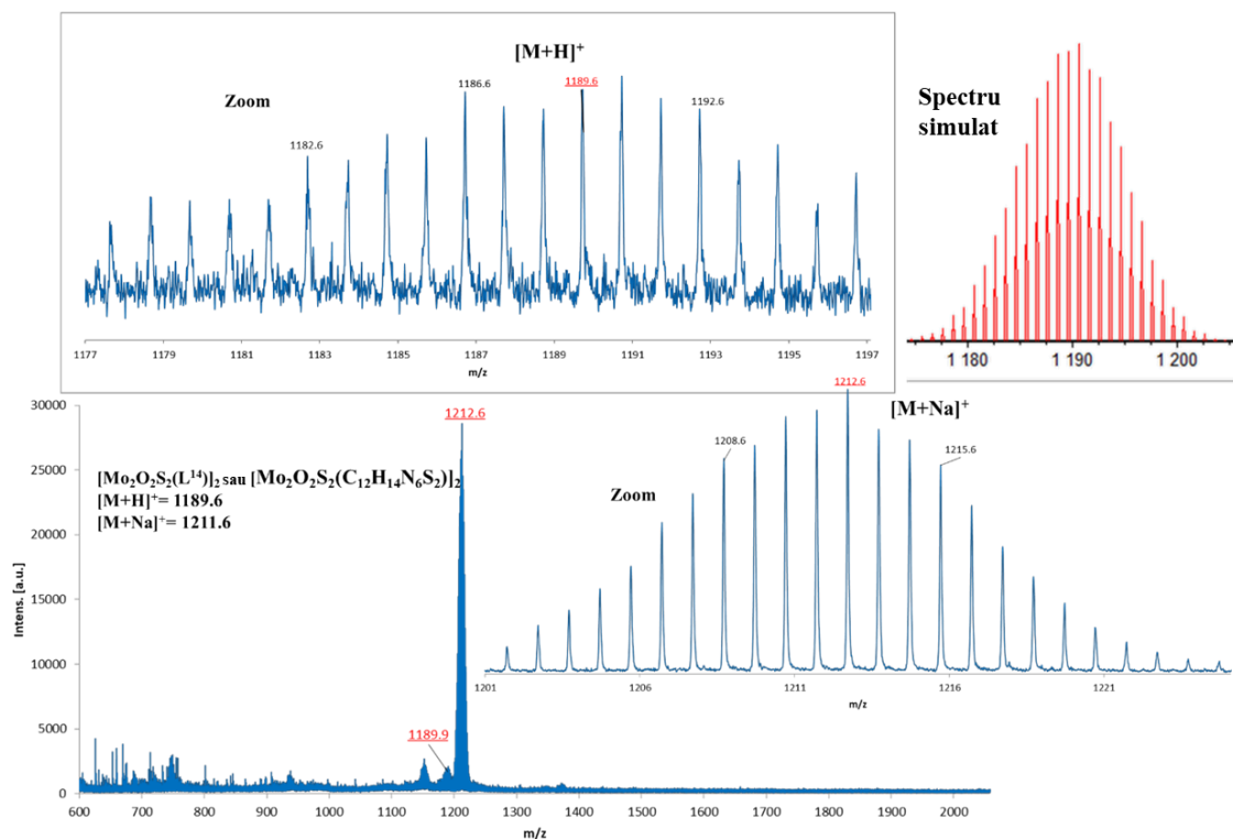
Fig. A6.7 Spectru de masă MALDI-TOF al compusului [Mo_2O_2S_2(L^{14})]_2
