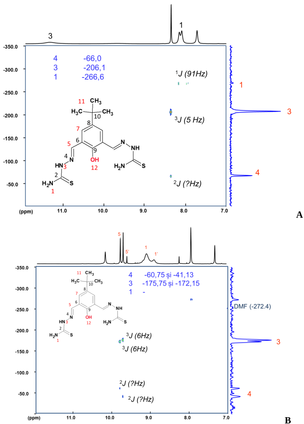
Fig. 4.26. 400 MHz ^1\text{H}\{^{15}\text{N}\} HMBC RMN ( \text{DMSO-d}_6 ) spectru al ligandului \text{H}_3\text{L}^{15} (A) și al complexului (B)
