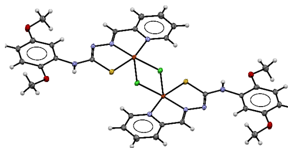
[Cu(L pa )Cl] 2 CCDC 1812640
