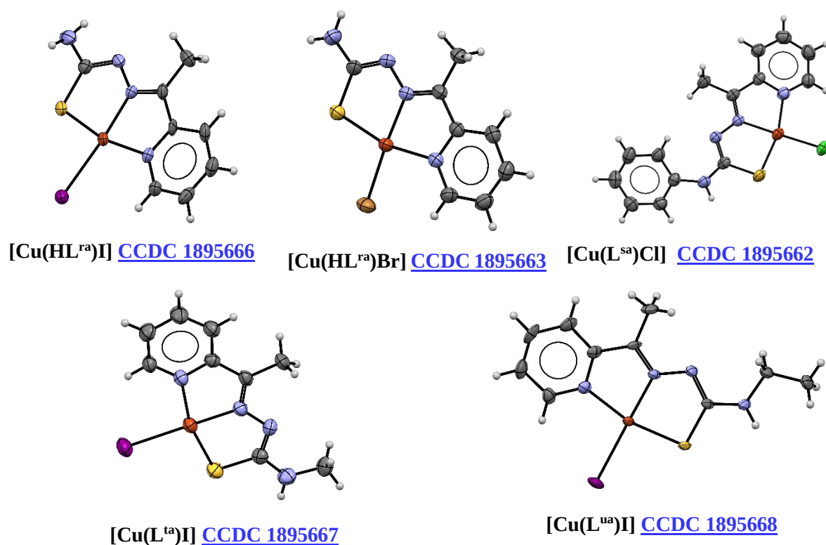
Fig. 1.19. Structura cristalină a compușilor studiați în baza Cu II [57]
