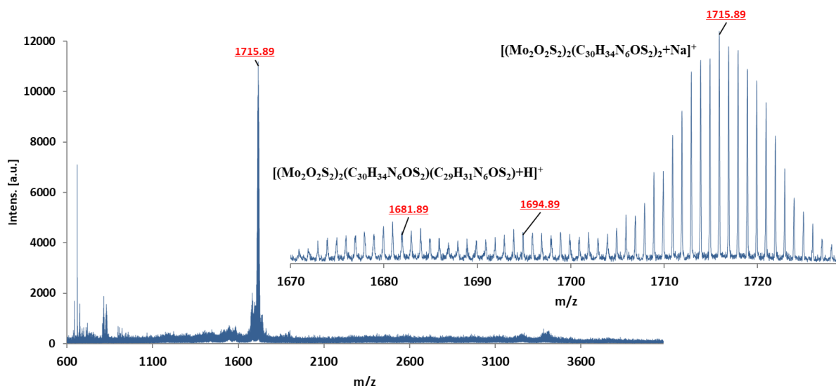
Fig. 4.19. Spectrul de masă MALDI-TOF al compusului [Mo_2O_2S_2(HL^{17})]_2
