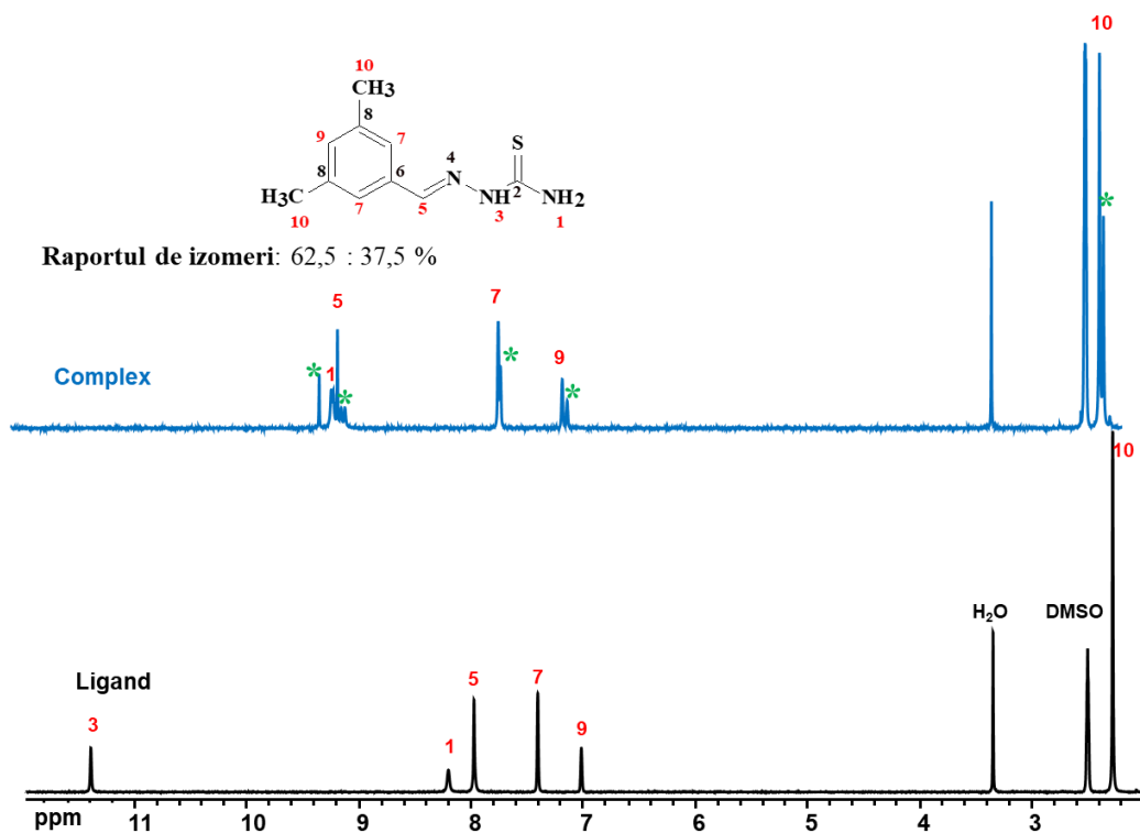
Fig. A4.2 300 MHz ^1\text{H} RMN (DMSO- \text{d}_6 ) spectru al ligandului \text{HL}^2 (negru) și al [\text{Mo}_2\text{O}_2\text{S}_2(\text{L}^2)_2] (albastru)
