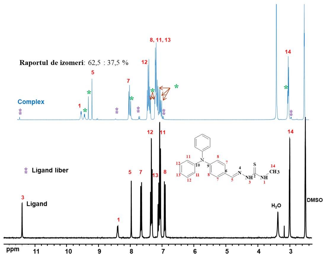
Fig. 3.10. 300 MHz 1 H RMN (DMSO-d 6 ) spectru al ligandului HL 5 (negru) și complexului [Mo 2 O 2 S 2 (L 5 ) 2 ] (albastru) (Pentru complex, atribuirile în roșu corespund izomerului de 62,5 %, în timp ce atribuirile în * corespund izomerului de 37,5 % și atribuirile în ** ligandului liber)
