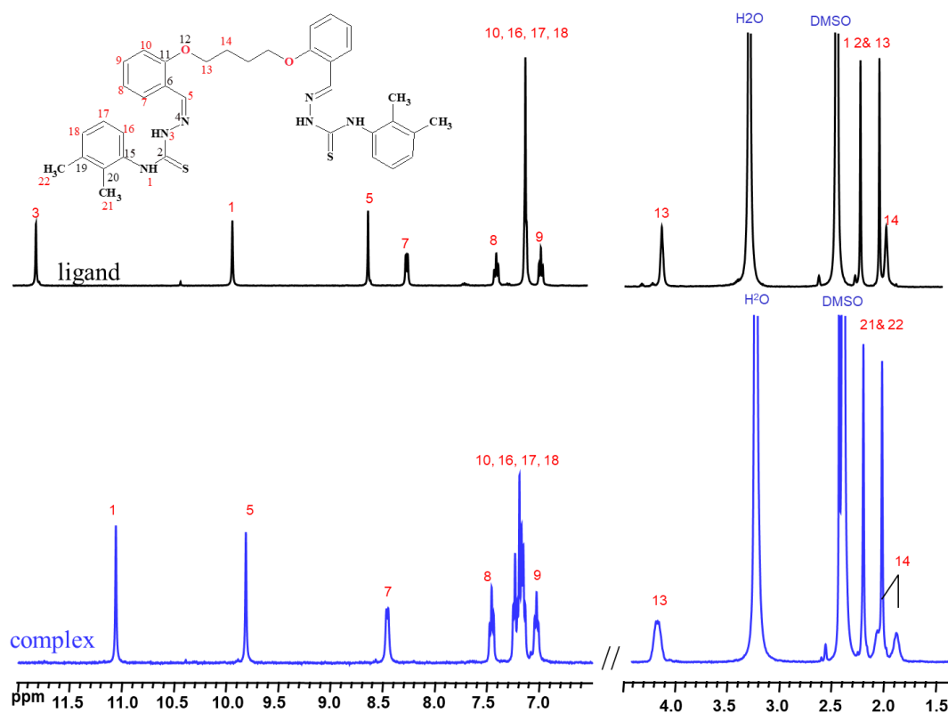
Fig. A8.1 400 MHz ^1\text{H} RMN ( \text{DMSO-d}_6 ) spectru al ligandului \text{H}_2\text{L}^7 (negru) și al [\text{Mo}_2\text{O}_2\text{S}_2(\text{L}^7)] (albastru)
