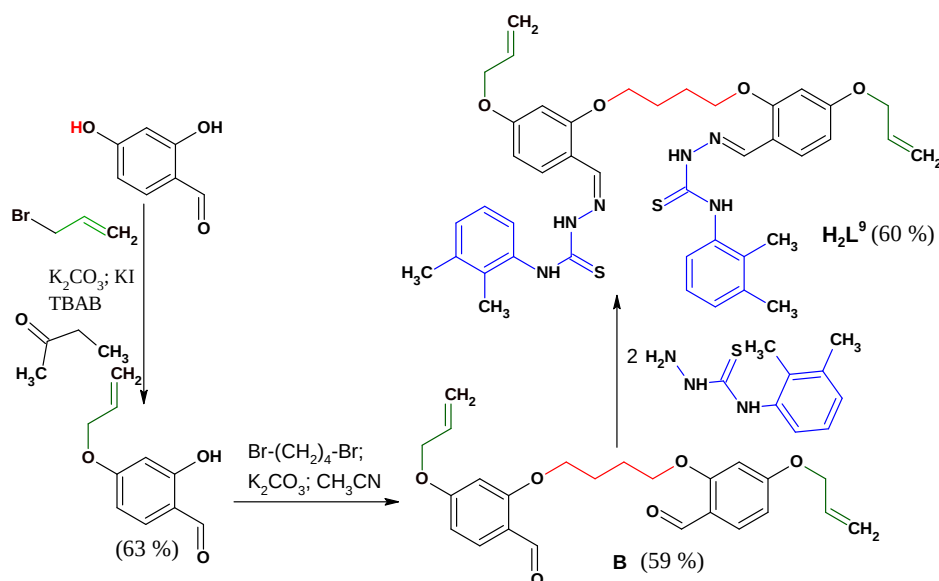
Fig. 2.3. Schema de sinteză a bis-tiosemicarbazonei \text{H}_2\text{L}^9
