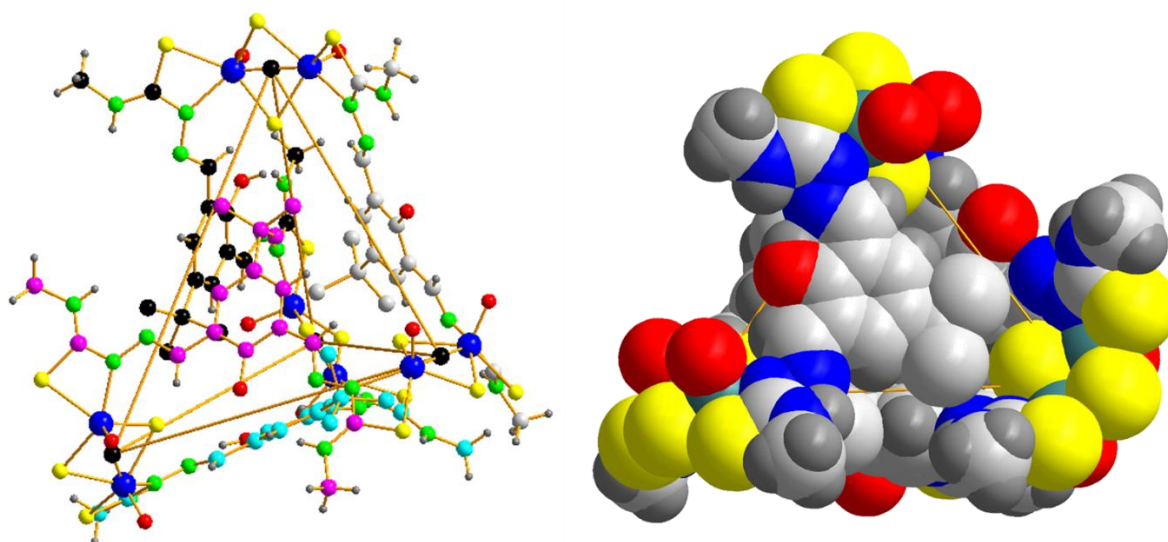
Fig. 4.20. Structura cristalografică a compusului [\text{Mo}_2\text{O}_2\text{S}_2(\text{HL}^{16})]_4 în model « ball and sticks » și în model Van der Waals
