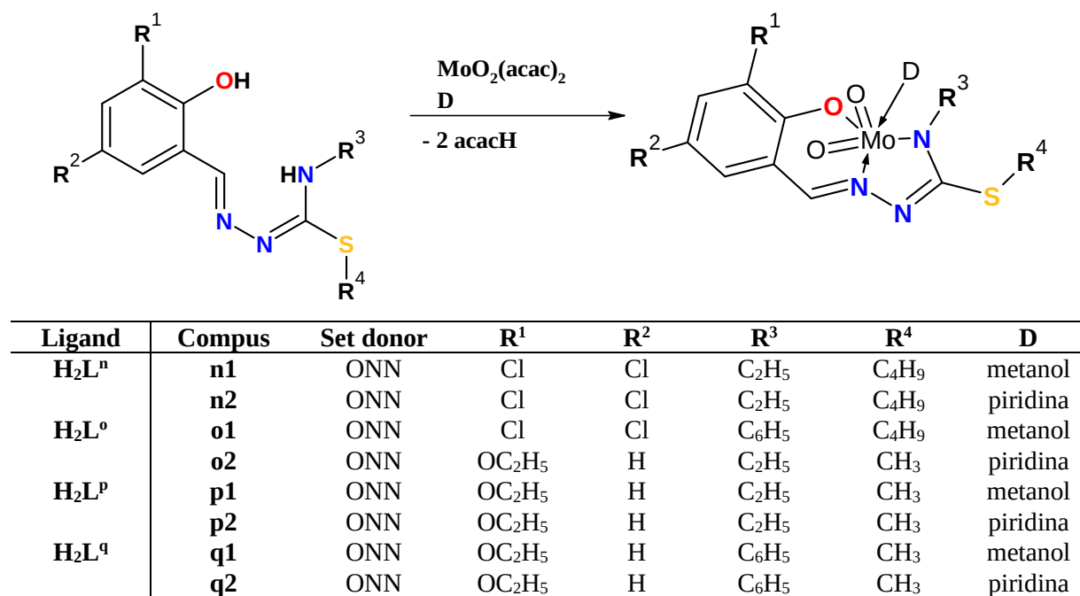
Fig. 1.8. Sinteza compușilor cis -oxomolibden în baza tiosemicarbazonelor H 2 L n-q [10]
