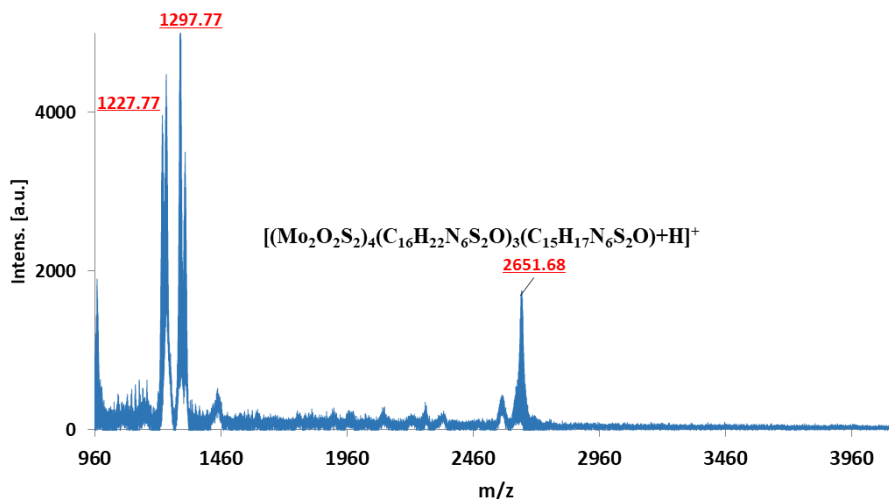
Fig. 4.17. Spectrul de masă MALDI-TOF al compusului [Mo_2O_2S_2(HL^{16})]_4
