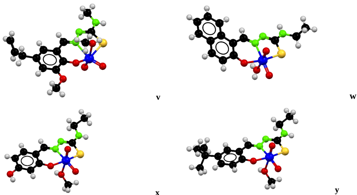
Fig. 1.10. Structurile cristaline ale compușilor v-y ( CCDC 895506 , 905156 , 913192 , 913194 ) [44]
