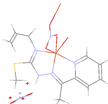
{[Cu(HL na )NO 3 ]NO 3 }_n CCDC 2046084
