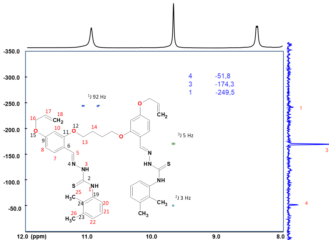
Fig. A10.6 400 MHz ^1H\{^{15}N\} HMBC RMN (DMSO- d_6 ) spectru al [Mo_2O_2S_2(L^9)]
