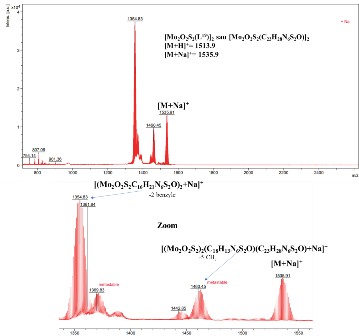
Fig. A6.10 Spectru de masă MALDI-TOF al compusului [\text{Mo}_2\text{O}_2\text{S}_2(\text{L}^{19})]_2
