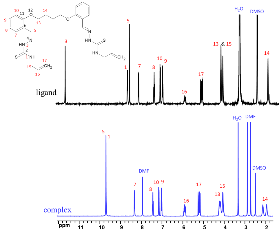
Fig. A8.2 400 MHz ^1\text{H} RMN ( \text{DMSO-d}_6 ) spectru al ligandului \text{H}_2\text{L}^8 (negru) și al [\text{Mo}_2\text{O}_2\text{S}_2(\text{L}^8)] (albastru)
