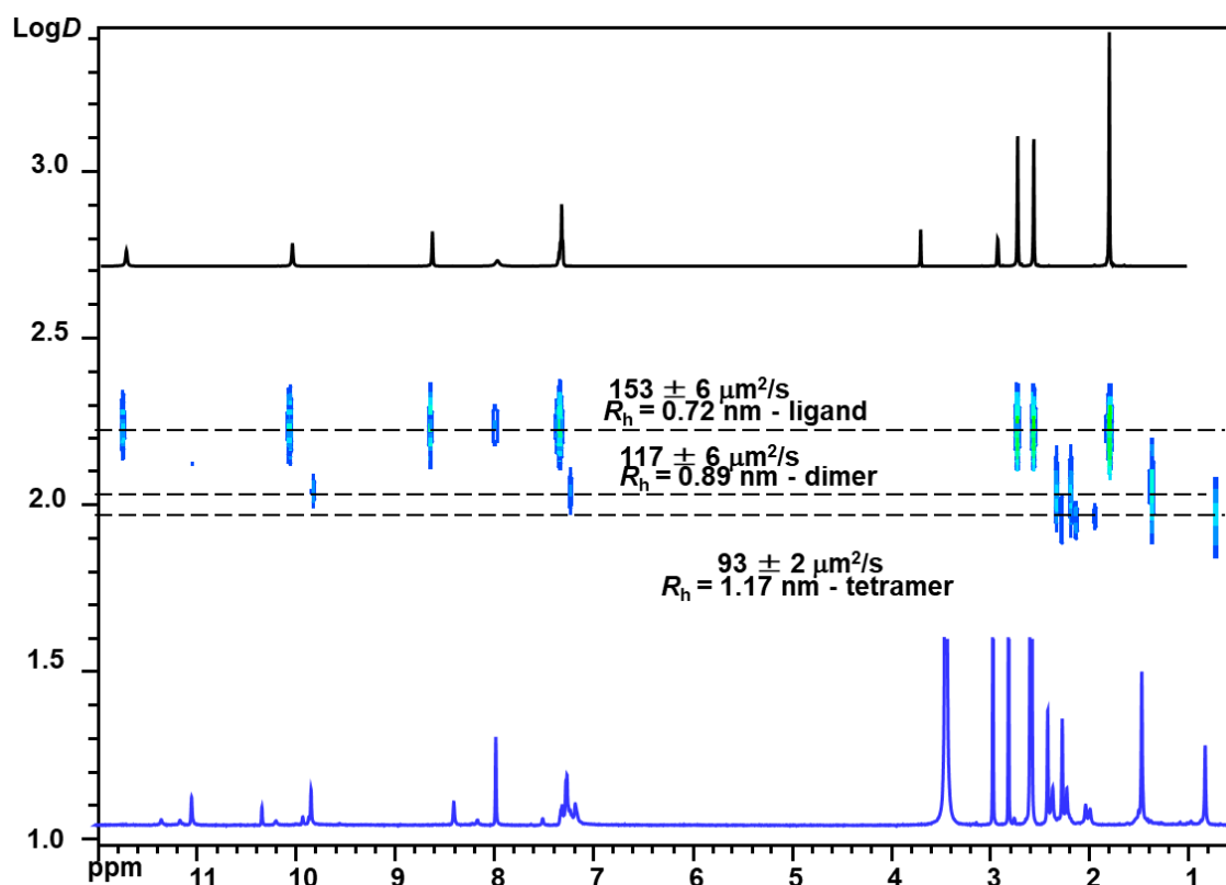
Fig. A9.9 400 MHz ^1\text{H} DOSY RMN ( \text{DMSO-d}_6 ) spectru al ligandului \text{H}_3\text{L}^{17} (negru) și al [\text{Mo}_2\text{O}_2\text{S}_2(\text{HL}^{17})]_2 și [\text{Mo}_2\text{O}_2\text{S}_2(\text{HL}^{17})]_4 (albastru)
