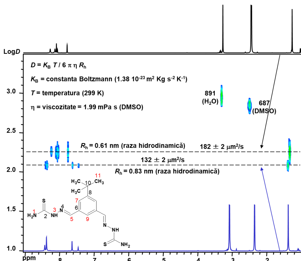
Fig. 4.9. Spectrele RMN ^1\text{H} DOSY (400 MHz, DMSO- d_6 ) ale ligandului \text{H}_2\text{L}^{11} (negru) și [\text{Mo}_2\text{O}_2\text{S}_2(\text{L}^{11})]_2 (albastru)
