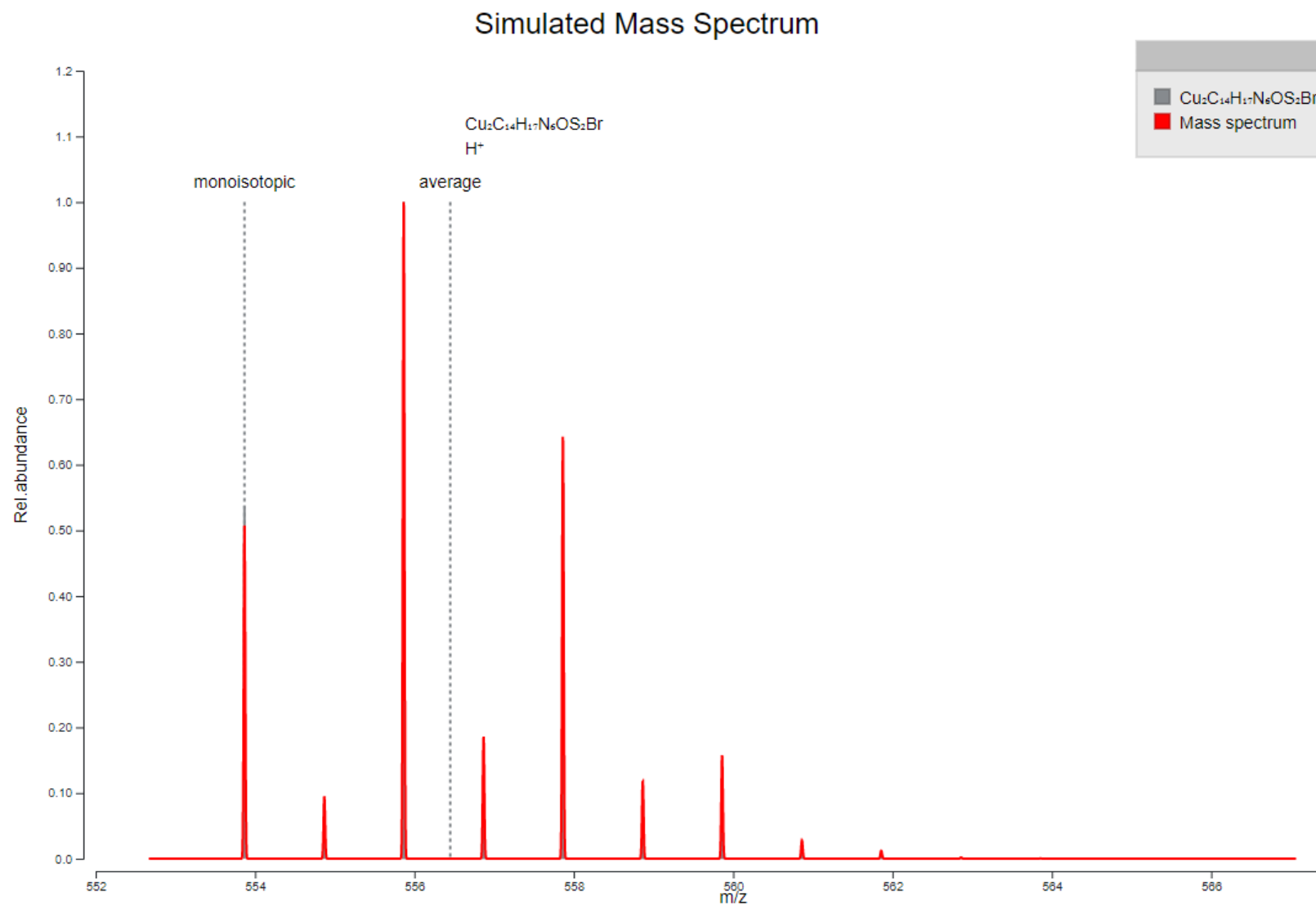
Fig. A6.13 Spectrul de masă simulat al compusului [\text{Cu}_2(\text{L}^{15})\text{Br}] prin Prot pi
