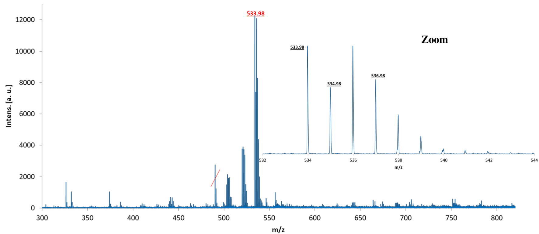
Fig. A6.20 Spectru de masă MALDI-TOF al compusului [\text{Cu}_2(\text{HL}^{16})\text{OCH}_3]\text{NO}_3
