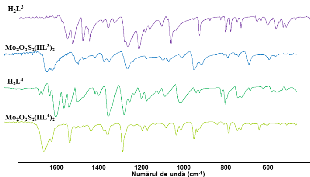
Fig. 3.5. Spectrele IR ale mono-tiosemicarbazonelor H_2L^3 , H_2L^4 și compușilor [Mo_2O_2S_2(HL^3)_2] și [Mo_2O_2S_2(HL^4)_2]
