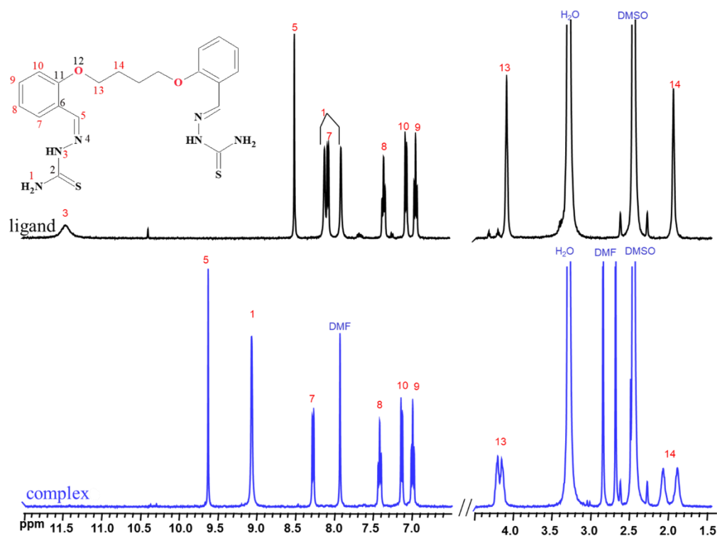
Fig. 4.6. 400 MHz 1 H RMN (DMSO-d 6 ) spectru al ligandului H 2 L 6 (negru) și al [Mo 2 O 2 S 2 (L 6 )] (albastru)
