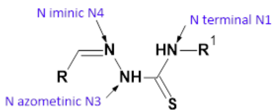
Tiosemicarbazone
