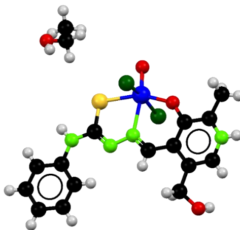
Fig. 1.3. Structura cristalină a compusului [MoOCl 2 (HL a )]·C 2 H 5 OH (ONS) CCDC 723346 [34]
