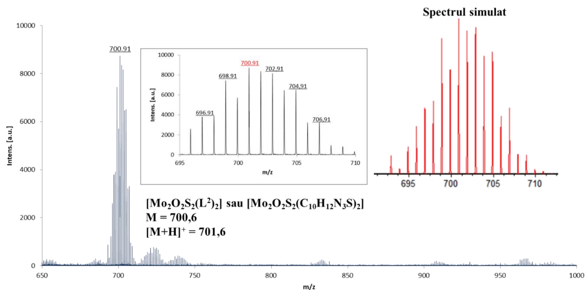
Fig. 3.6. Spectrul de masă MALDI-TOF al compusului [Mo 2 O 2 S 2 (C 10 H 12 N 3 S) 2 ]
