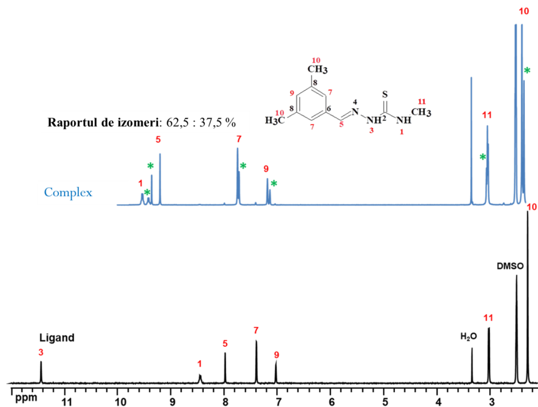
Fig. A4.1 300 MHz ^1\text{H} RMN (DMSO- \text{d}_6 ) spectru al ligandului \text{HL}^1 (negru) și al [\text{Mo}_2\text{O}_2\text{S}_2(\text{L}^1)_2] (albastru)
