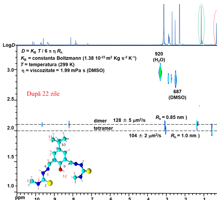
Fig. 4.24. 400 MHz ^1\text{H} DOSY RMN (DMSO- d_6 ) spectrul amestecului după 22 de zile
