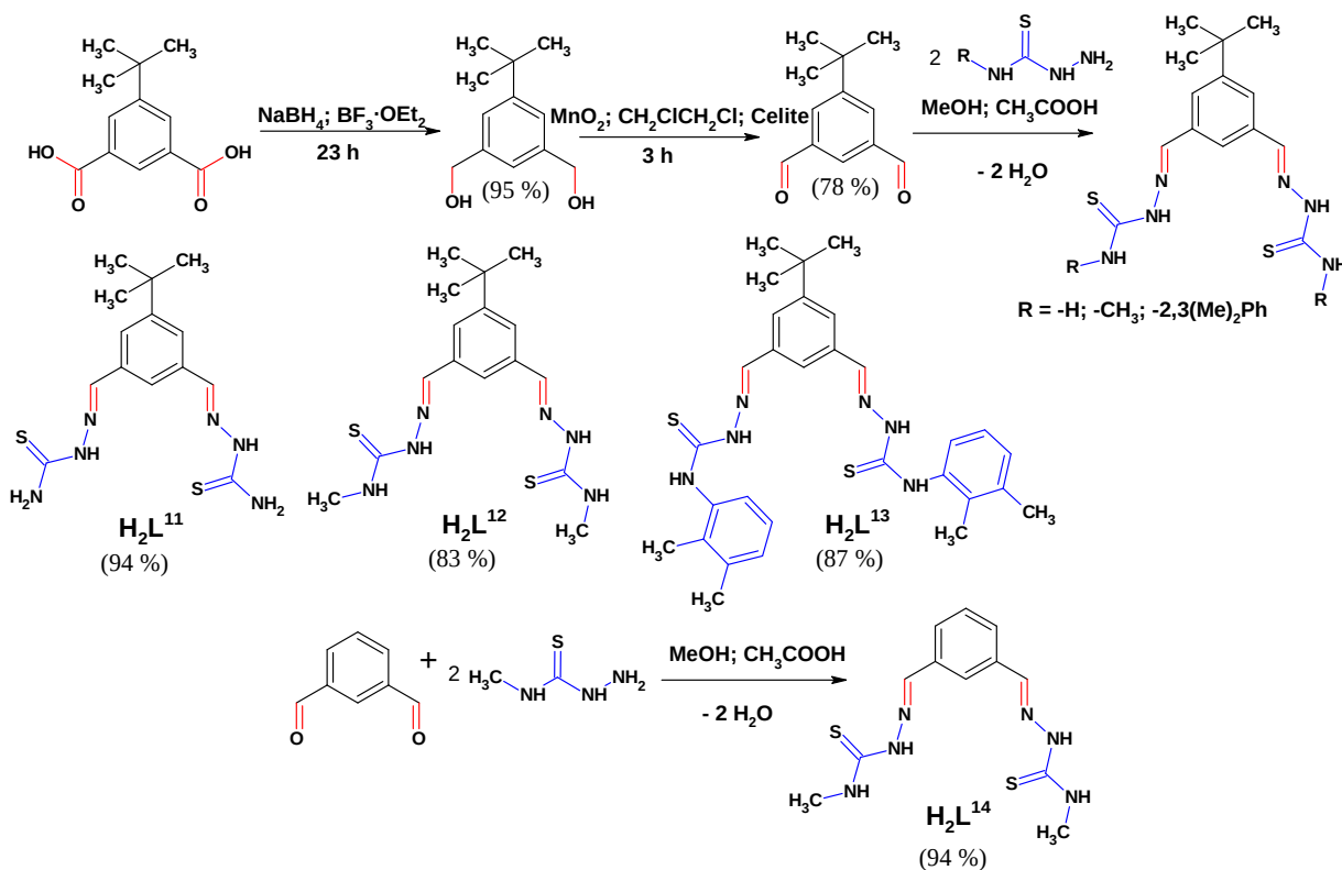
Fig. 2.5. Schema de sinteză a bis-tiosemicarbazonelor H 2 L 11-14
