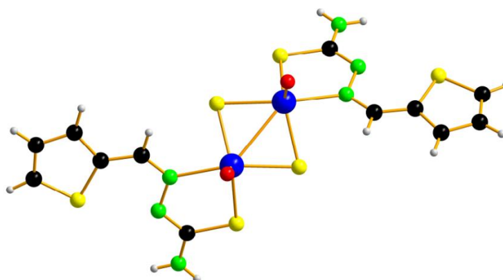
Izomerul trans
