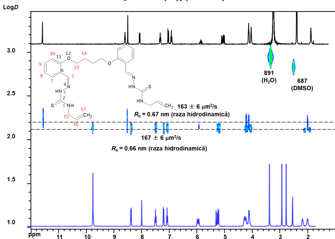
Fig. A9.2 400 MHz ^1\text{H} DOSY RMN ( \text{DMSO-d}_6 ) spectru al ligandului \text{H}_2\text{L}^8 (negru) și al [\text{Mo}_2\text{O}_2\text{S}_2(\text{L}^8)] (albastru)
