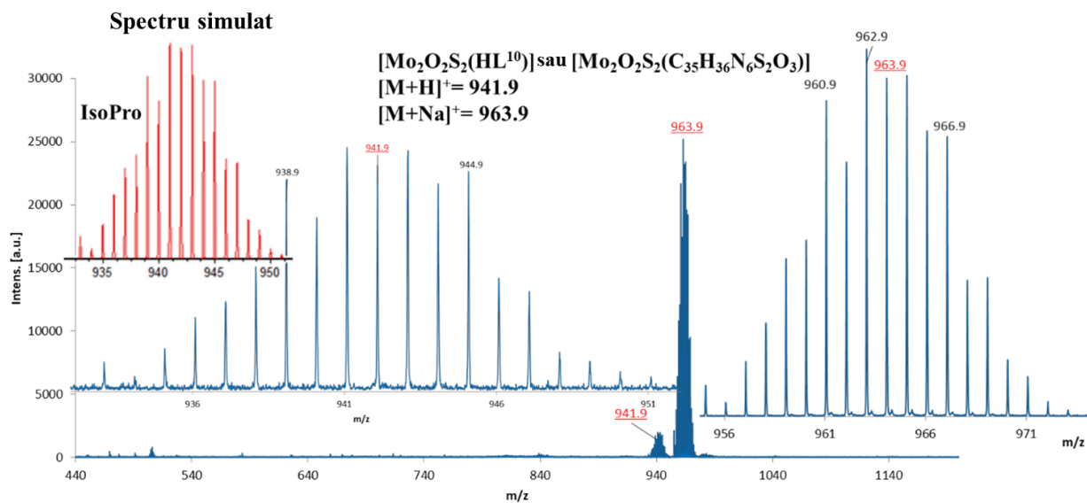
Fig. A6.4 Spectru de masă MALDI-TOF al compusului [\text{Mo}_2\text{O}_2\text{S}_2(\text{HL}^{10})]
