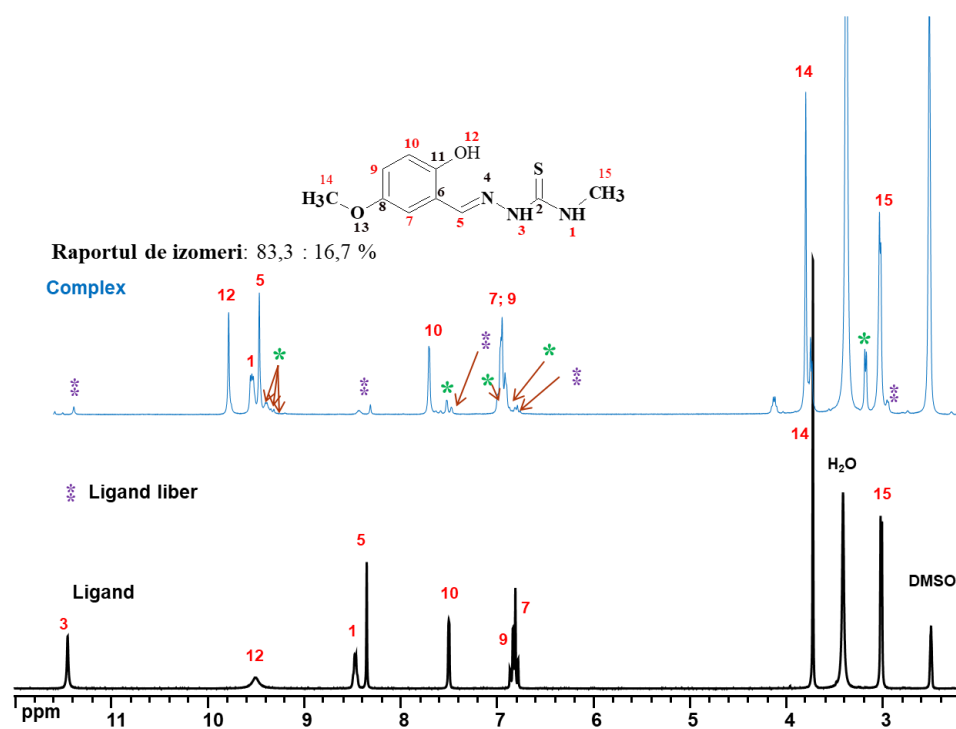
Fig. A4.3 300 MHz ^1\text{H} RMN (DMSO- d_6 ) spectru al ligandului \text{H}_2\text{L}^4 (negru) și al [\text{Mo}_2\text{O}_2\text{S}_2(\text{HL}^4)_2] (albastru)
