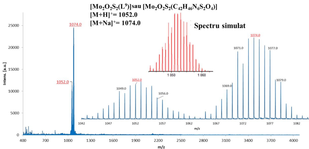
Fig. A6.3 Spectru de masă MALDI-TOF al compusului [Mo 2 O 2 S 2 (L 9 )]
