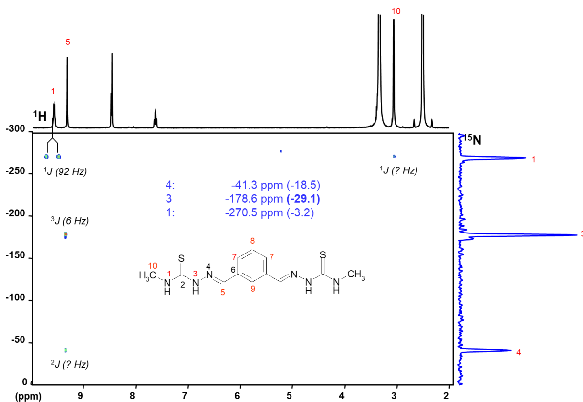
Fig. A10.13 400 MHz ^1H\{^{15}N\} HMBC RMN (DMSO- d_6 ) spectru al [Mo_2O_2S_2(L^{14})]_2
