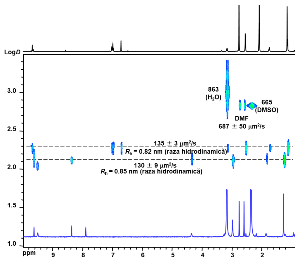
Fig. A9.11 400 MHz ^1\text{H} DOSY RMN (DMSO- \text{d}_6 ) spectru al ligandului \text{H}_4\text{L}^{20} (negru) și al [(\text{Mo}_2\text{O}_2\text{S}_2)_2\text{L}^{20}] (albastru)
