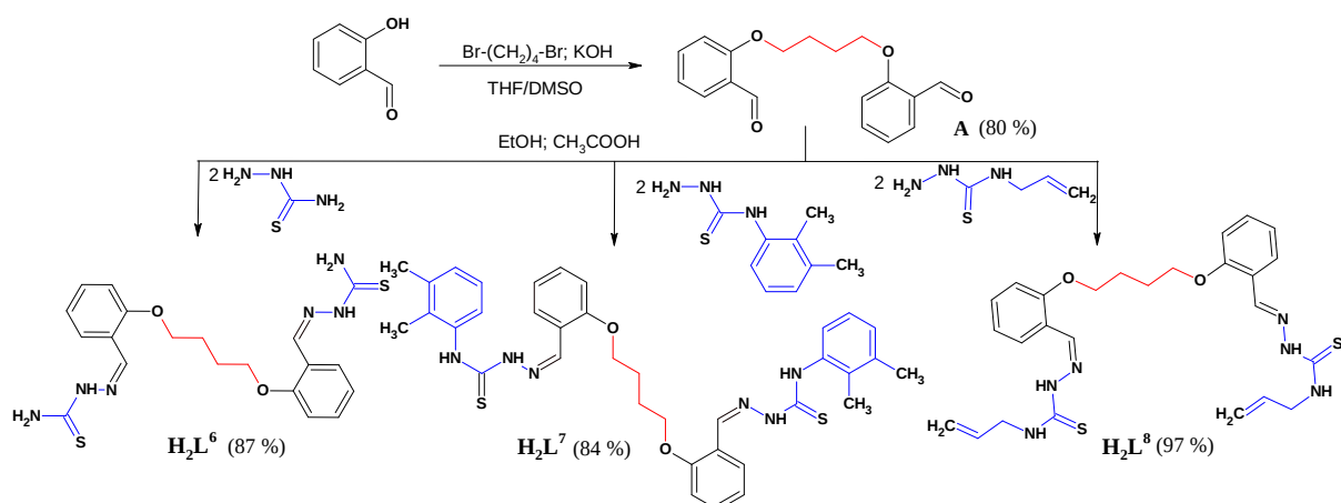
Fig. 2.2. Schema de sinteză a bis-tiosemicarbazonelor flexibile \text{H}_2\text{L}^{6-8}
