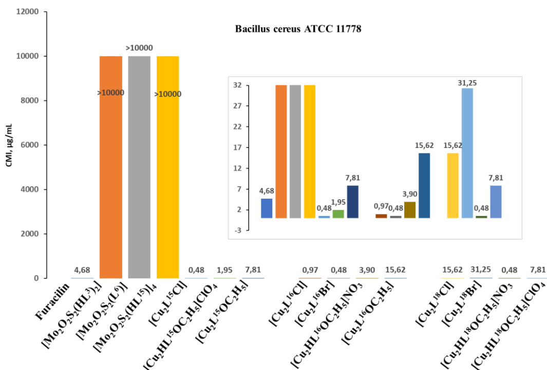
Fig. 5.3. Activitatea antimicrobiană a compușilor față de Bacillus cereus ATCC 11778
