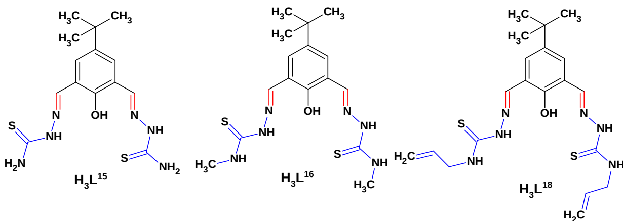
Fig. 4.29. Structurile fenol bis-tiosemicarbazonelor H 3 L 15-16,18 sintetizate
