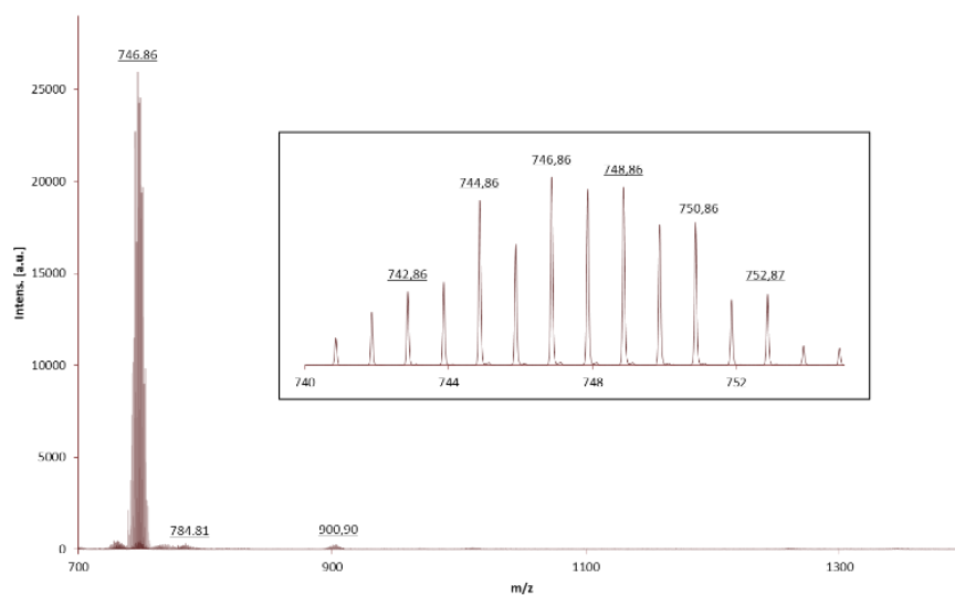
Fig. 3.3. Spectru de masă MALDI-TOF al complexului [\text{Mo}_2\text{O}_2\text{S}_2(\text{C}_{11}\text{H}_9\text{N}_4\text{S})_2] (B)
