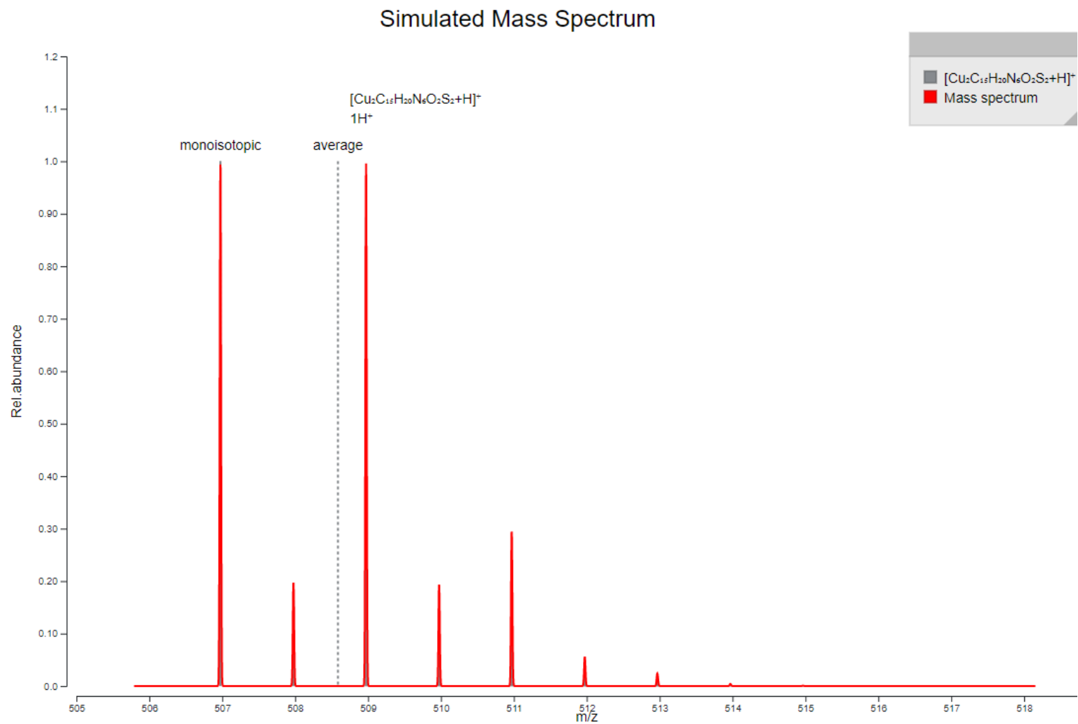
Fig. A6.17 Spectrul de masă simulat al compusului [\text{Cu}_2(\text{HL}^{15})\text{OCH}_3]^+\text{ClO}_4^- prin Prot pi
