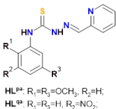
Fig. 1.18. Structura generală a tiosemicarbazonelor HL pa-qa și structura cristalină a complexului [Cu(L pa )Cl] 2 [56]
