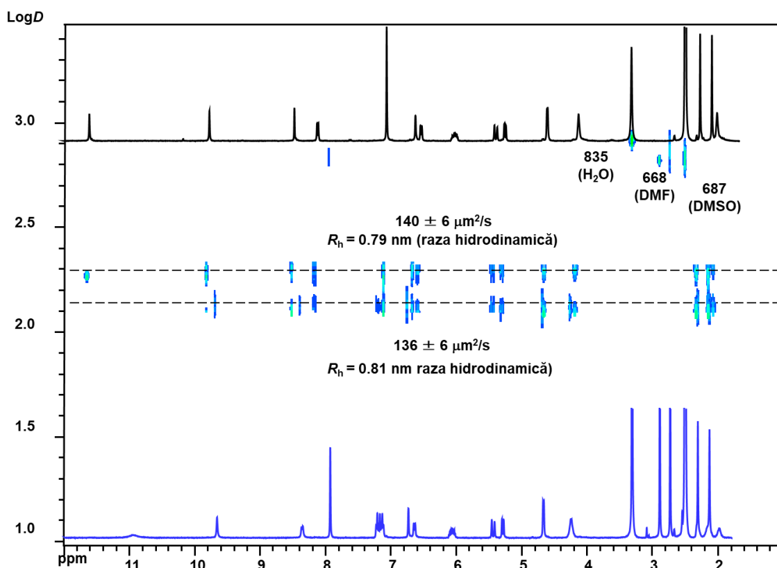
Fig. A9.3 400 MHz ^1\text{H} DOSY RMN (DMSO- d_6 ) spectru al ligandului \text{H}_2\text{L}^9 (negru) și al [\text{Mo}_2\text{O}_2\text{S}_2(\text{L}^9)] (albastru)
