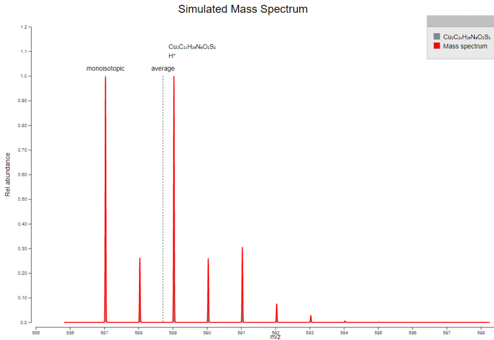
Fig. A6.29 Spectrul de masă simulat al compusului [\text{Cu}_2(\text{HL}^{18})\text{OCH}_3]^+\text{NO}_3^- prin Prot pi
