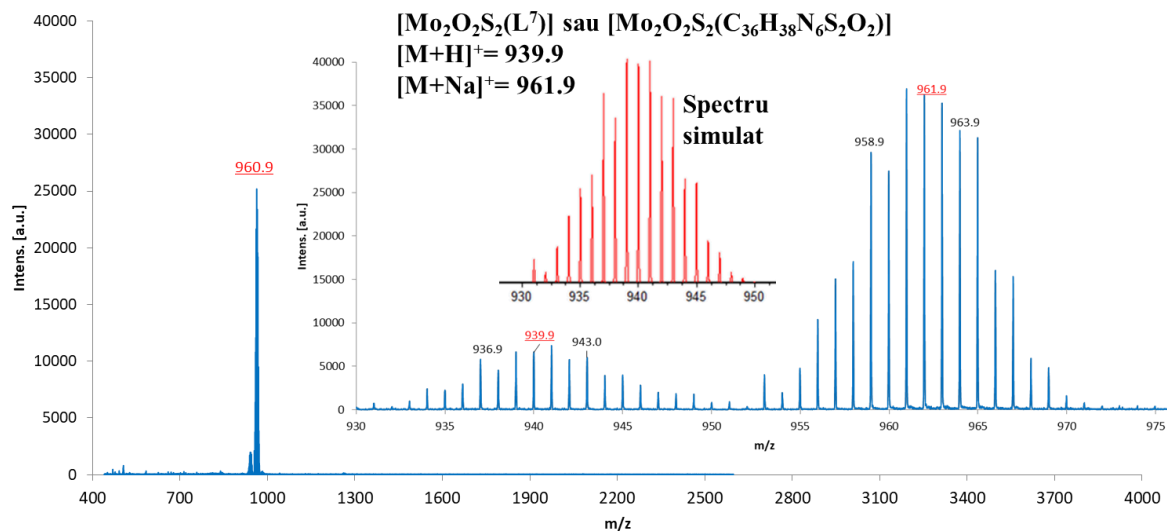
Fig. A6.1 Spectru de masă MALDI-TOF al compusului [Mo 2 O 2 S 2 (L 7 )]
