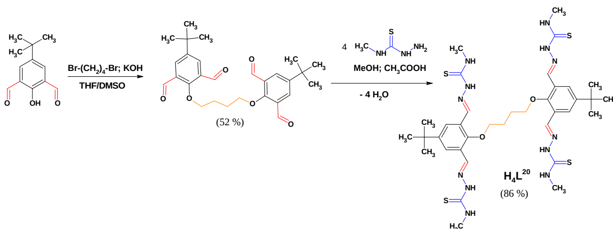
Fig. 2.8. Schema de sinteză a tetrakis-tiosemicarbazonei \text{H}_4\text{L}^{20}
