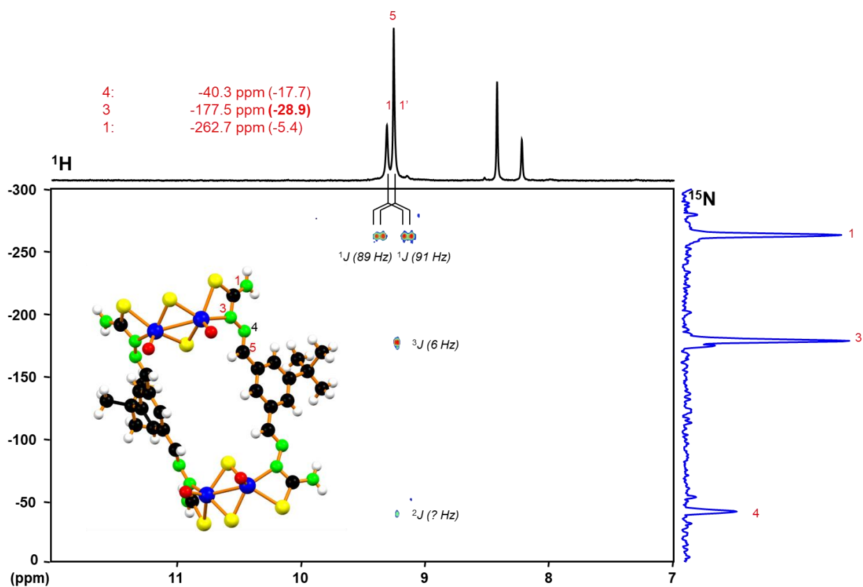
Fig. 4.14. Spectrul RMN 400 MHz ^1\text{H}\{^{15}\text{N}\} HMBC al complexului [\text{Mo}_2\text{O}_2\text{S}_2(\text{L}^{11})]_2 în \text{DMSO-d}_6
