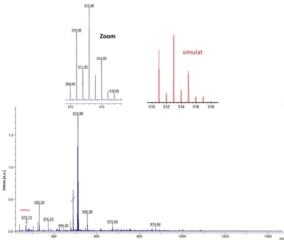
Fig. 4.31 Spectrul de masă MALDI-TOF al compusului [\text{Cu}_2(\text{L}^{15})\text{Cl}]
