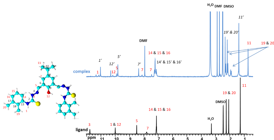
Fig. 4.25. 400 MHz ^1\text{H} RMN ( \text{DMSO-d}_6 ) spectrul ligandului \text{H}_3\text{L}^{17} (negru) și complexului (albastru, atribuirile cu negru corespund speciei dimer și cu roșu speciei tetramer)
