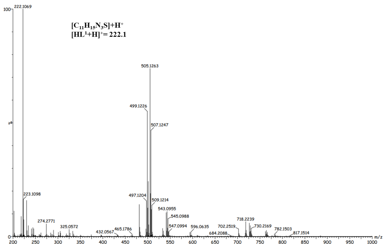
Fig. A2.1 Spectru de masă ESI-MS al mono-tiosemicarbazonei HL 1
