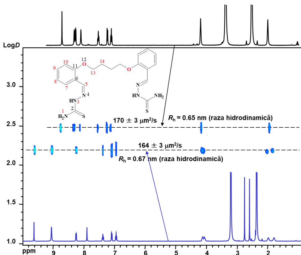
Fig. 4.8. Spectrele RMN ^1\text{H} DOSY (400 MHz, DMSO- d_6 ) ale ligandului \text{H}_2\text{L}^6 (negru) și [\text{Mo}_2\text{O}_2\text{S}_2(\text{L}^6)] (albastru)
