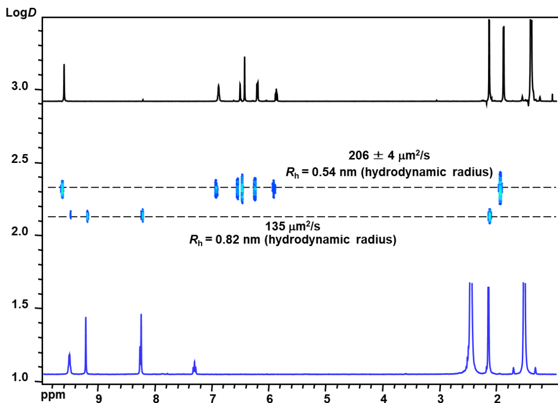
Fig. A9.7 400 MHz ^1\text{H} DOSY RMN (DMSO- \text{d}_6 ) spectru al ligandului \text{H}_2\text{L}^{14} (negru) și al [\text{Mo}_2\text{O}_2\text{S}_2(\text{L}^{14})_2] (albastru)
