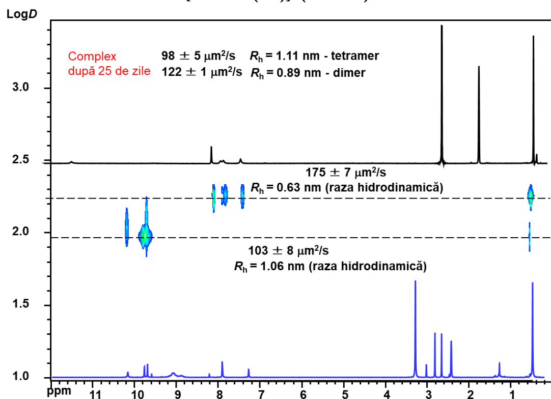
Fig. A9.8 400 MHz ^1\text{H} DOSY RMN (DMSO- \text{d}_6 ) spectru al ligandului \text{H}_3\text{L}^{15} (negru) și al [\text{Mo}_2\text{O}_2\text{S}_2(\text{HL}^{15})_2] și [\text{Mo}_2\text{O}_2\text{S}_2(\text{HL}^{15})_4] (albastru)
