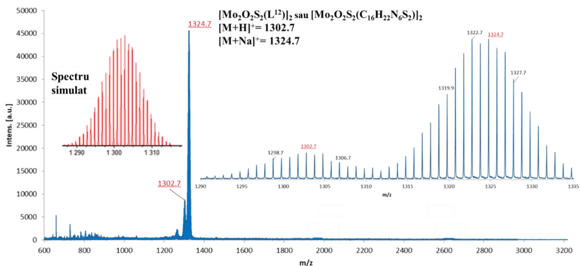
Fig. A6.5 Spectru de masă MALDI-TOF al compusului [\text{Mo}_2\text{O}_2\text{S}_2(\text{L}^{12})]_2
