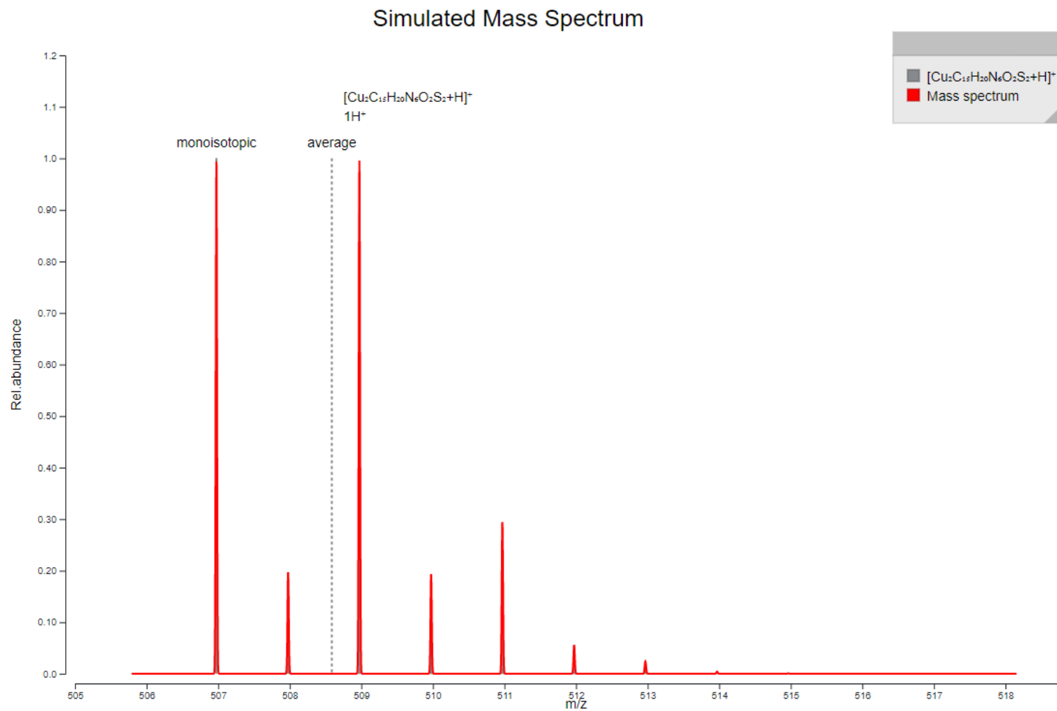
Fig. A6.15 Spectrul de masă simulat al compusului [\text{Cu}_2(\text{HL}^{15})\text{OCH}_3]^+\text{NO}_3^- prin Prot pi
