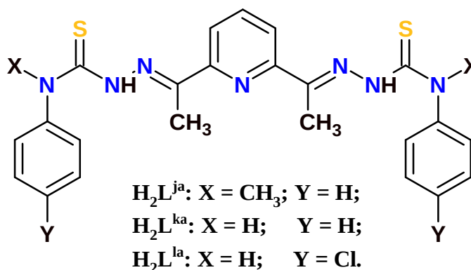
Fig. 1.14. Structura generală a bis-tiosemicarbazonelor H_2L^{ja-la} [50]
