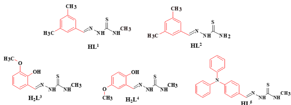
Fig. 3.4. Structurile chimice ale mono-tiosemicarbazonelelor \text{HnL}^{1-5} ( n = 1 - 2 )
