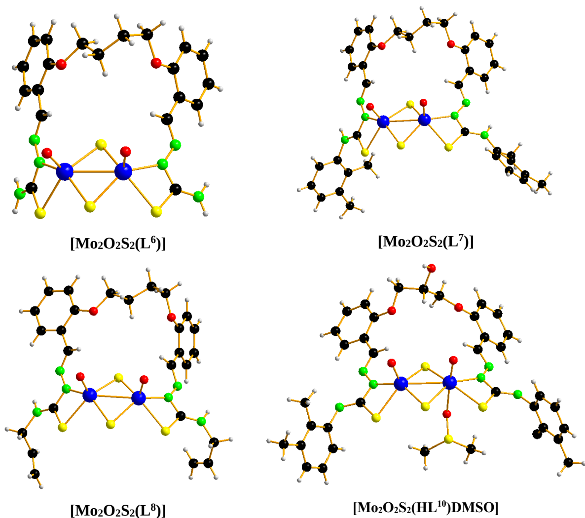
Fig. 4.4. Structurile moleculare ale compușilor sintetizați cu liganzi flexibili: [Mo 2 O 2 S 2 (L 6 )], [Mo 2 O 2 S 2 (L 7 )], [Mo 2 O 2 S 2 (L 8 )] și [Mo 2 O 2 S 2 (HL 10 )DMSO]
