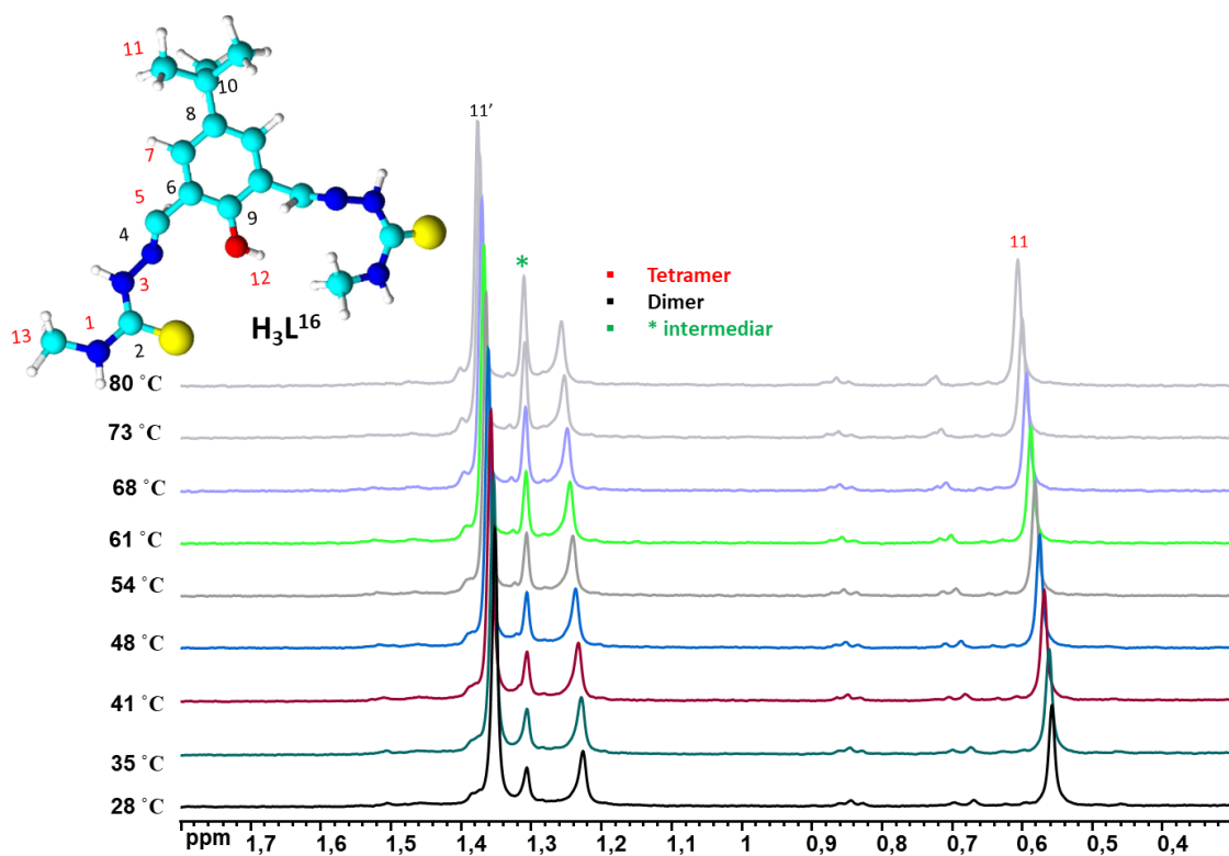
Fig. A8.11 400 MHz ^1\text{H} RMN (DMSO- d_6 ) spectru al complexului [\text{Mo}_2\text{O}_2\text{S}_2(\text{HL}^{16})]_2 și [\text{Mo}_2\text{O}_2\text{S}_2(\text{HL}^{16})]_4 la diferite temperaturi (de la 80 la 28 °C)
