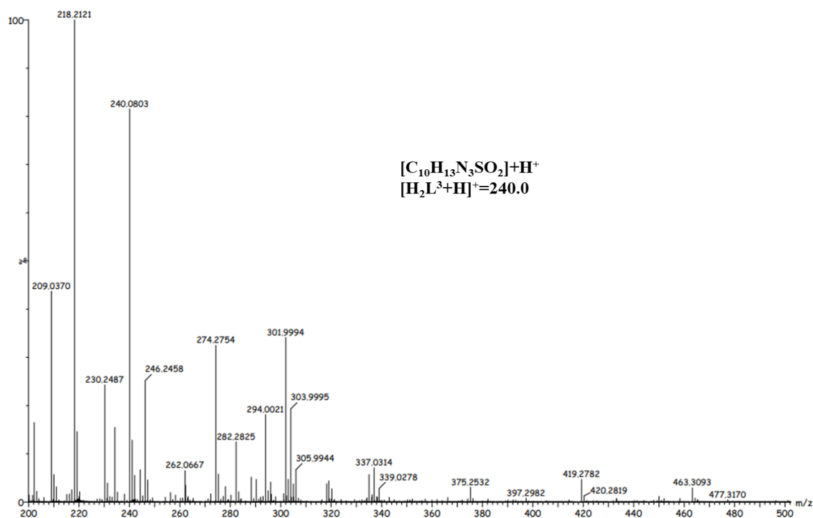
Fig. A2.3 Spectru de masă ESI-MS al mono-tiosemicarbazonei H_2L^3
