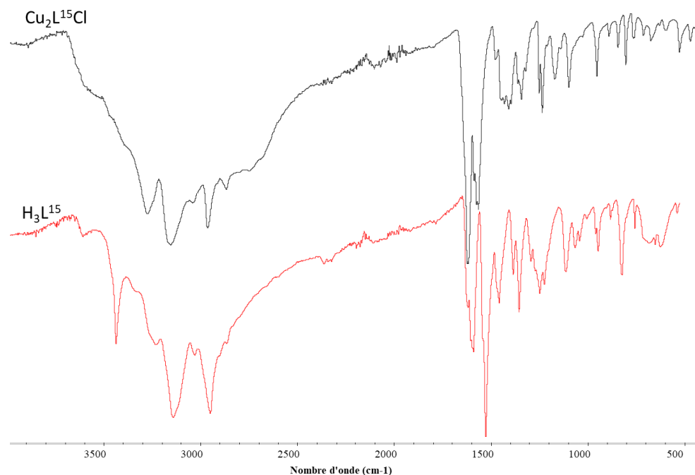
Fig. 4.30. Spectrele IR ale bis-tiosemicarbazonei H 3 L 15 și compusului [Cu 2 (L 15 )Cl]
