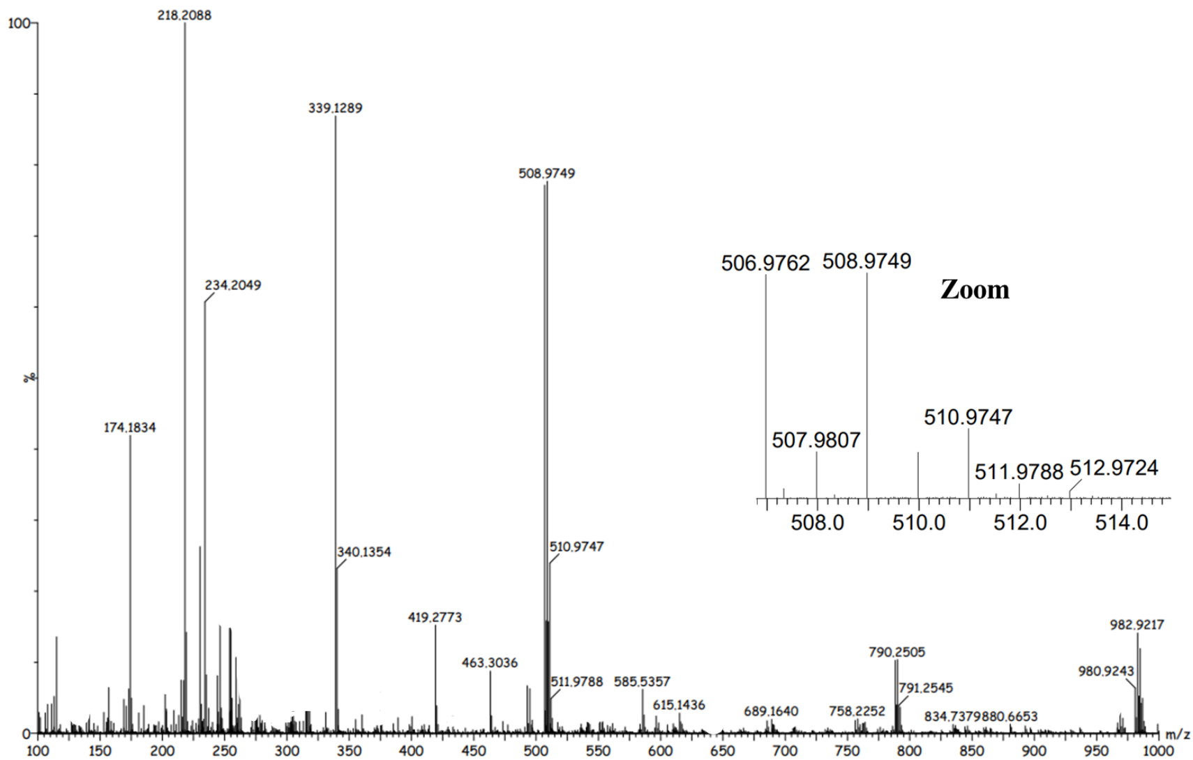
Fig. A6.16 Spectru de masă ESI-MS al compusului [\text{Cu}_2(\text{HL}^{15})\text{OCH}_3]^+\text{ClO}_4^-
