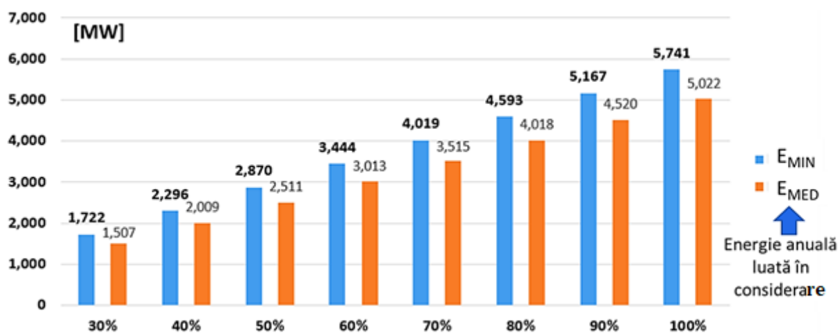
Figura 1. Necesarul de putere în CEF pentru diverse niveluri de acoperire anuală a consumului în Republica Moldova
