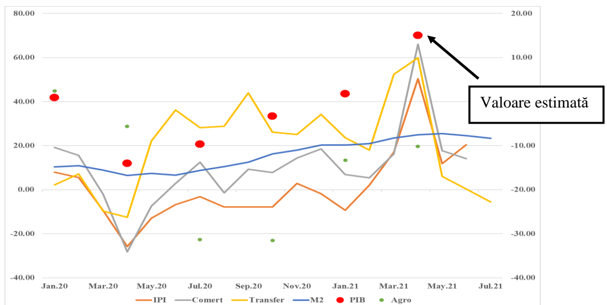
Figura 3.2. Indicator operativ pentru creșterea economică și a variabilelor exogene în R. Moldova, % (frecvență lunară, PIB (scala dreapta))
