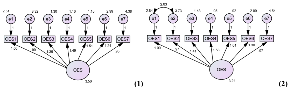
Figura 3.1. Potrivirea modelelor factoriale al scalei OES-RO: (1) modelul primar; (2) – modelul secundar după corelarea erorilor pentru itemul 1 și 2 a OES-RO
